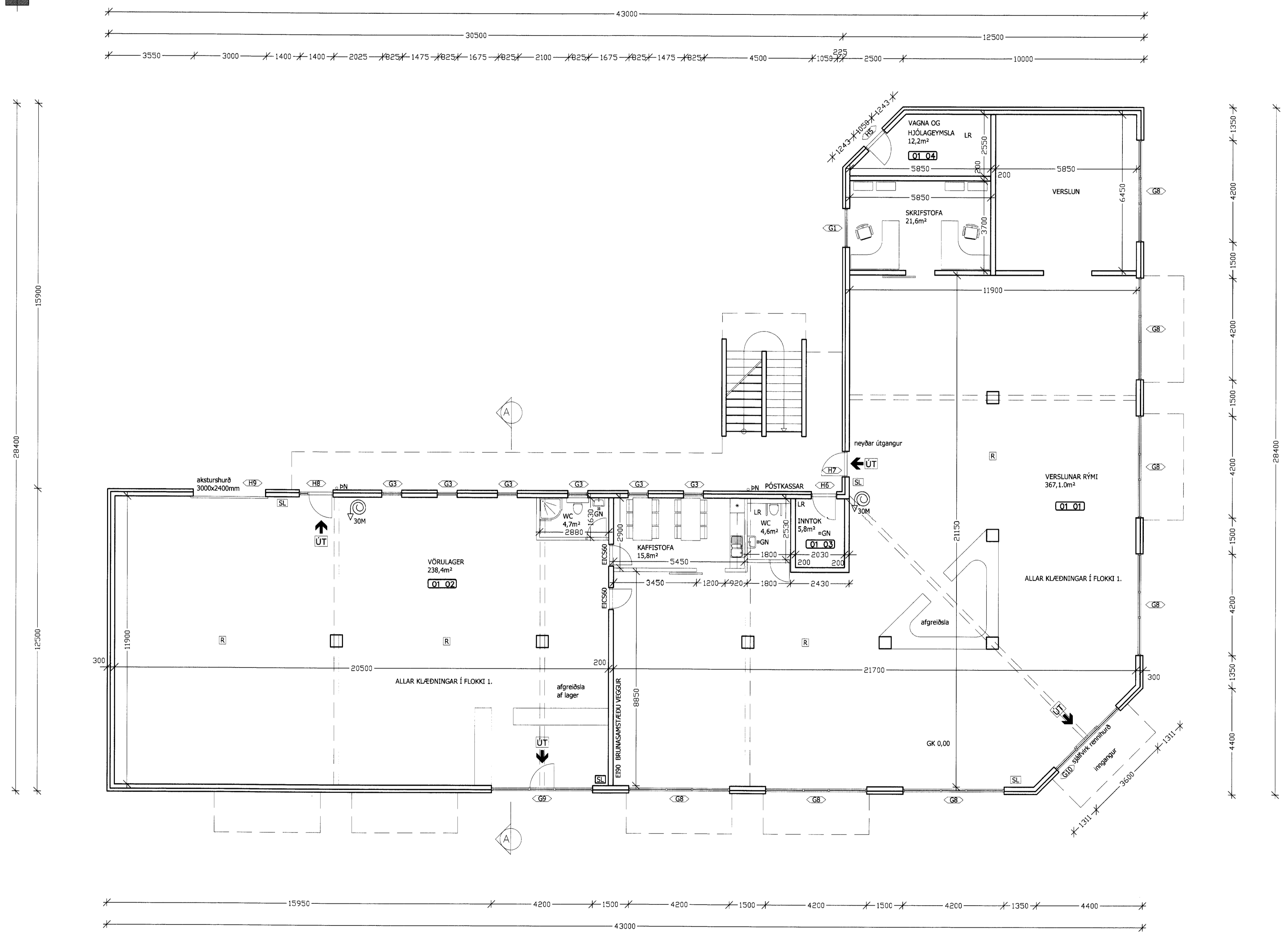
GRUNNMYND 2.HÆÐ 1:100
