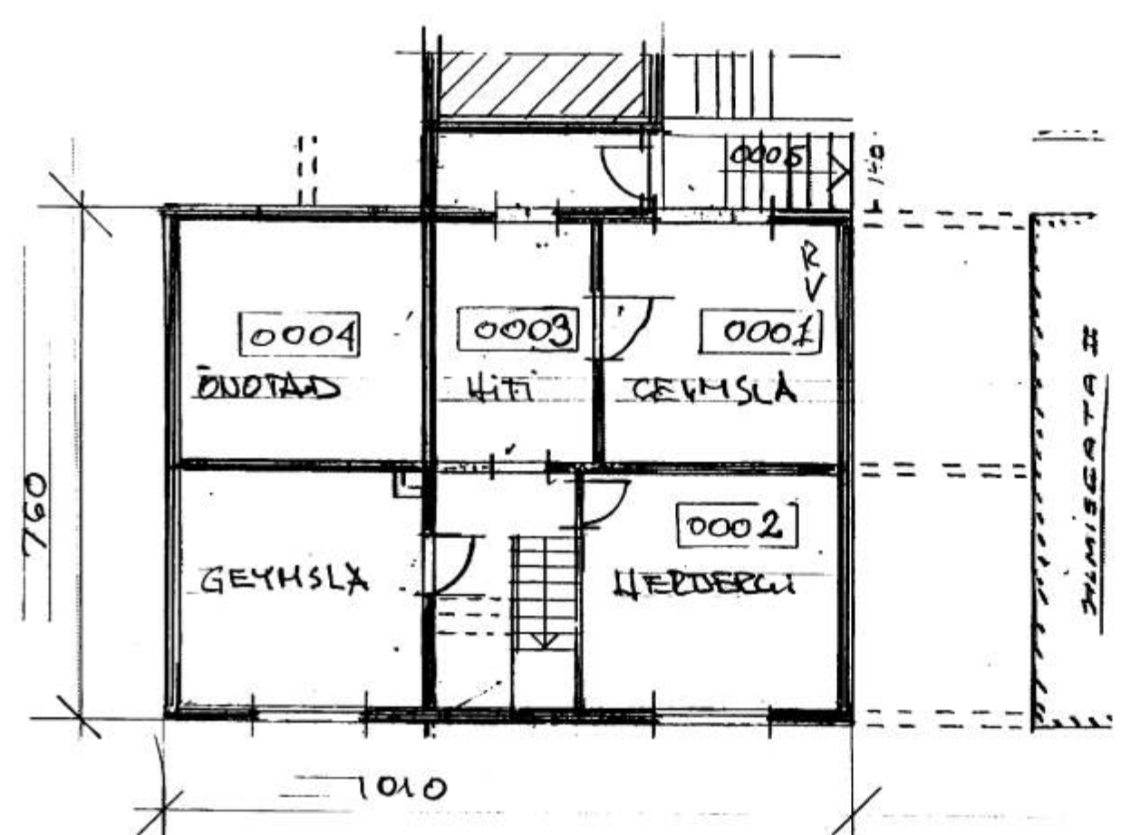
GRUNNMYND KJALLARI
