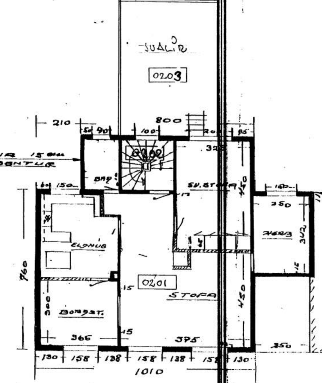
GRUNNMYND 2. HÆÐ
