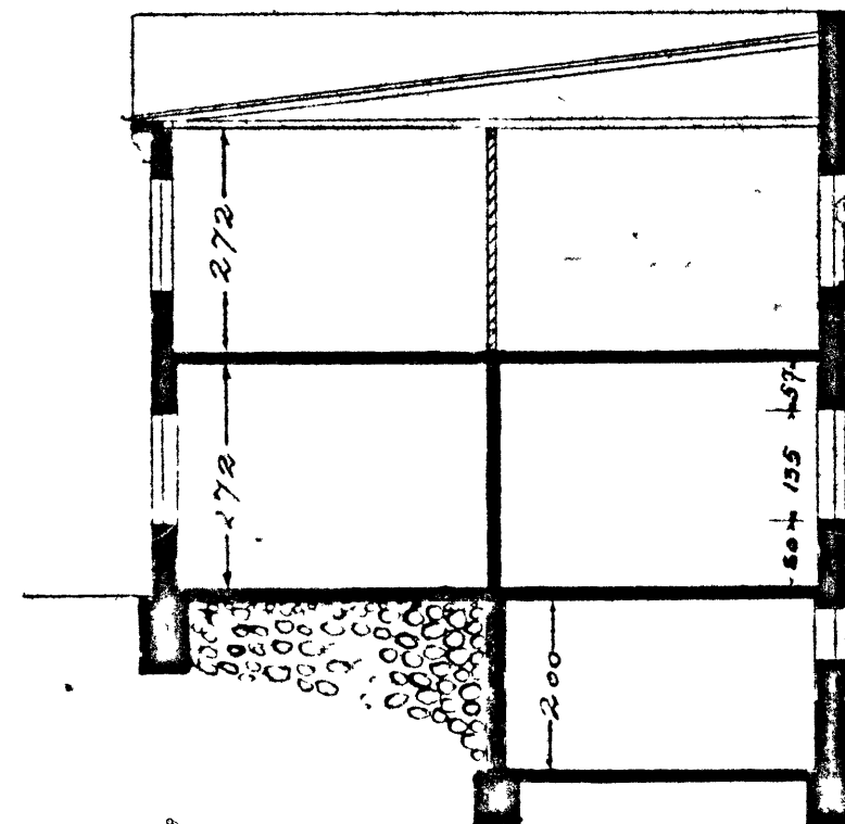
Sneiðing
