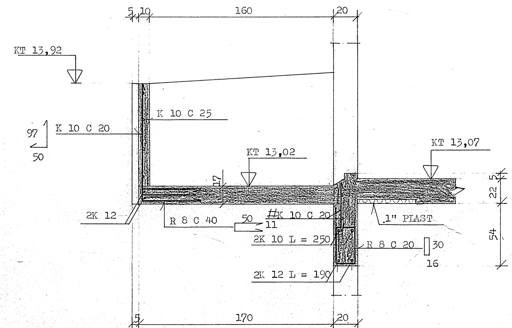
SNID B - B. 1:20.
