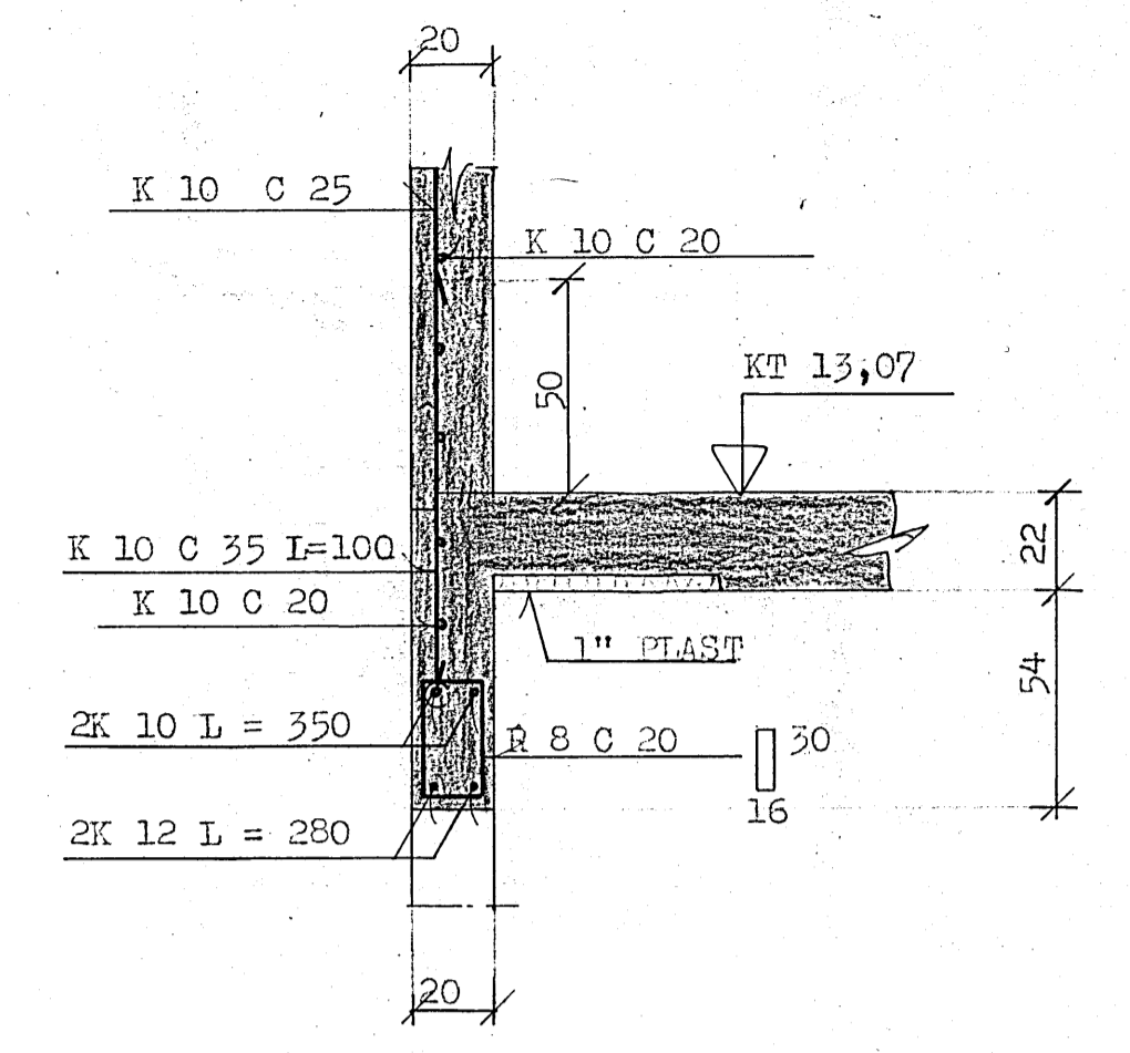
SNID B - B. 1:20.
