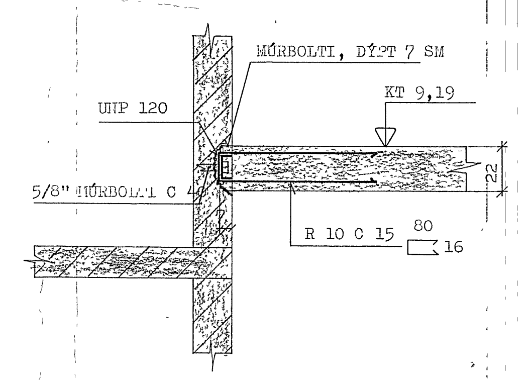
SNID D-D 1:20
