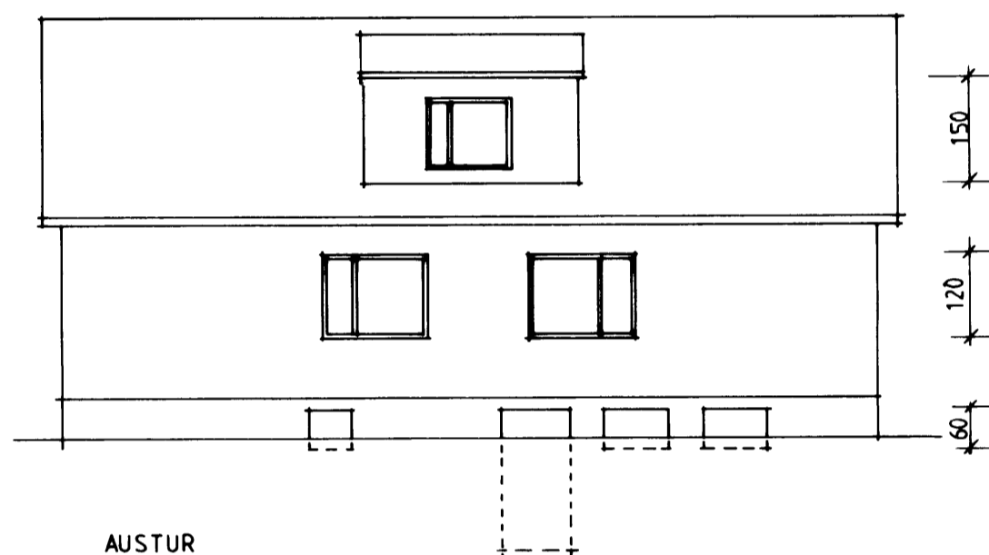
AUSTUR
