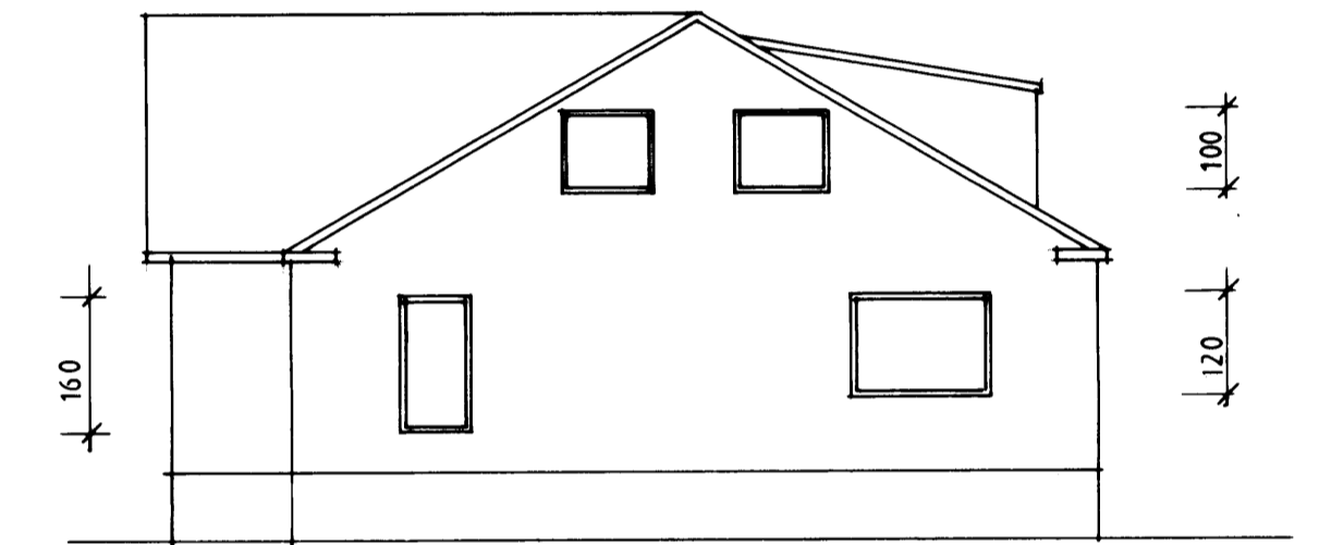
SÜÐUR
