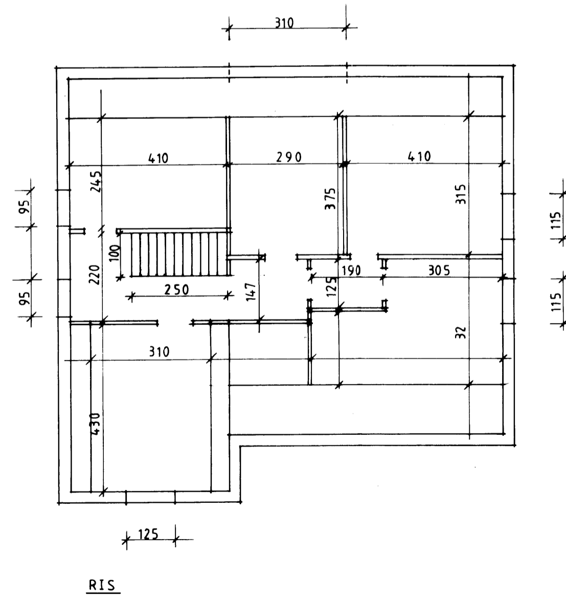
RIS
