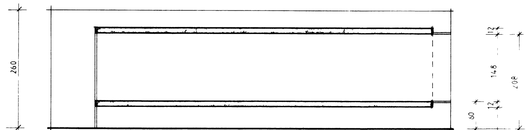
NORÐURVEGGUR
