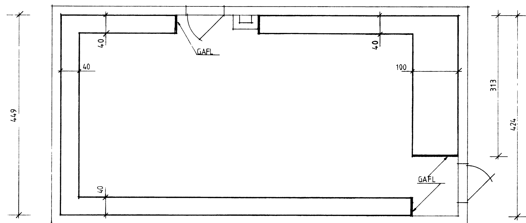
GRNNMYND 1:50
