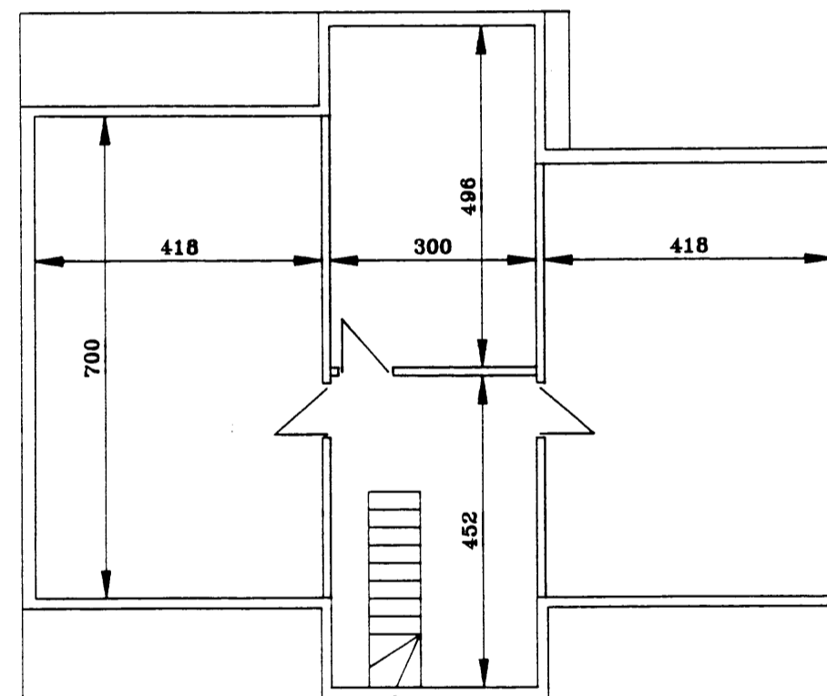
Breyting
