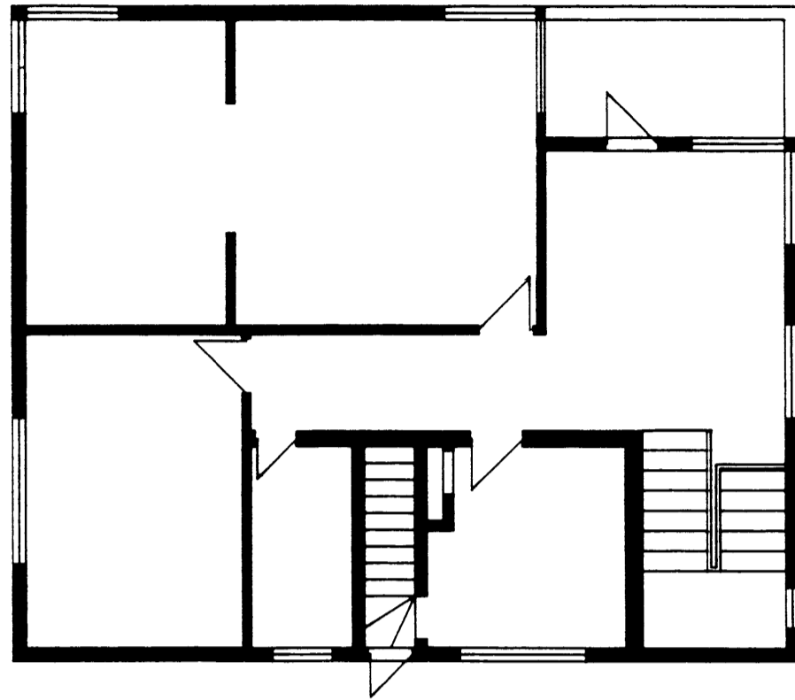
1. hæð
