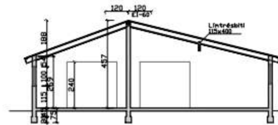
SNID A-A
