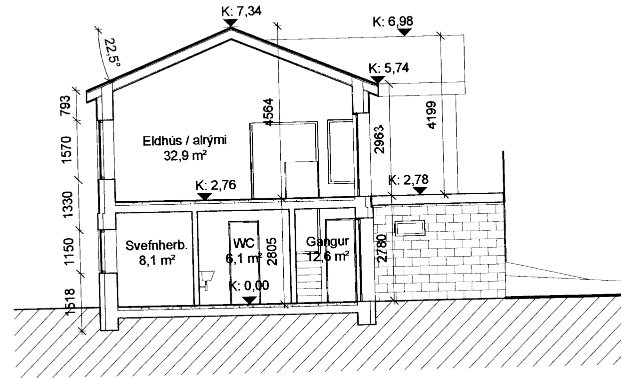
A-A 1 : 100
