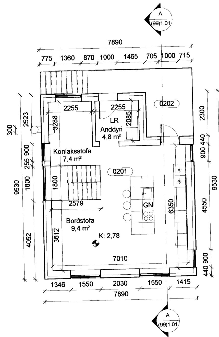
Grunnmynd, 2. hæð 1 : 100
