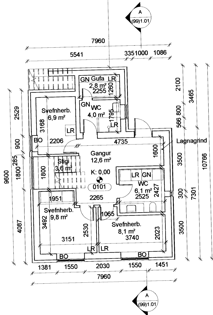
Grunnmynd, 1. hæð 1 : 100
