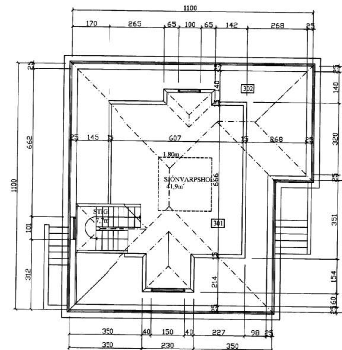
GRUNNMYND 2. HÆÐ
