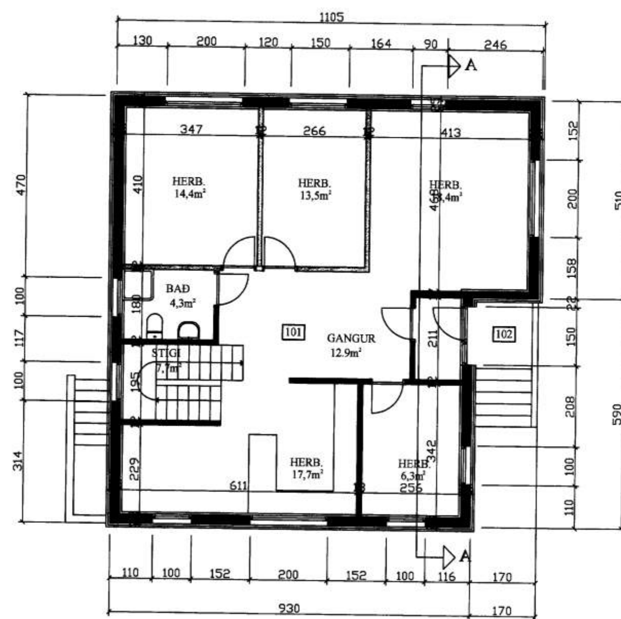
GRUNNMYND 1. HÆÐ
