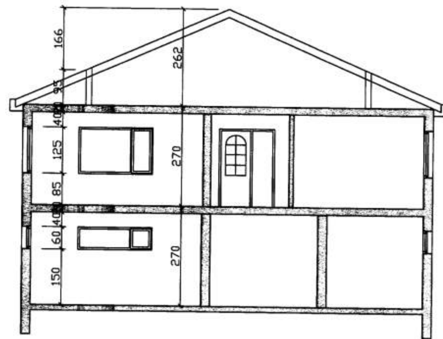
SNID A-A
