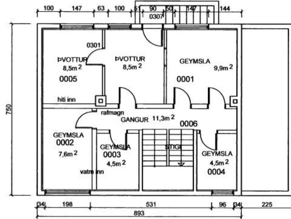
GRUNNMYND KJALLARI
