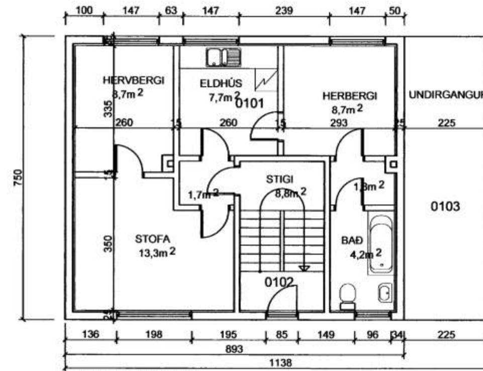
GRUNNMYND 1. HÆÐ
