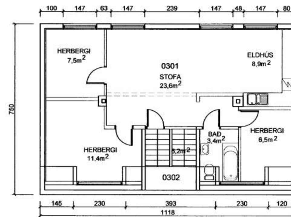
GRUNNMYND RIS
