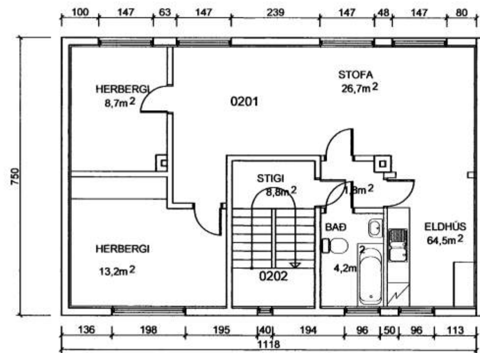
GRUNNMYND 2. HÆÐ
