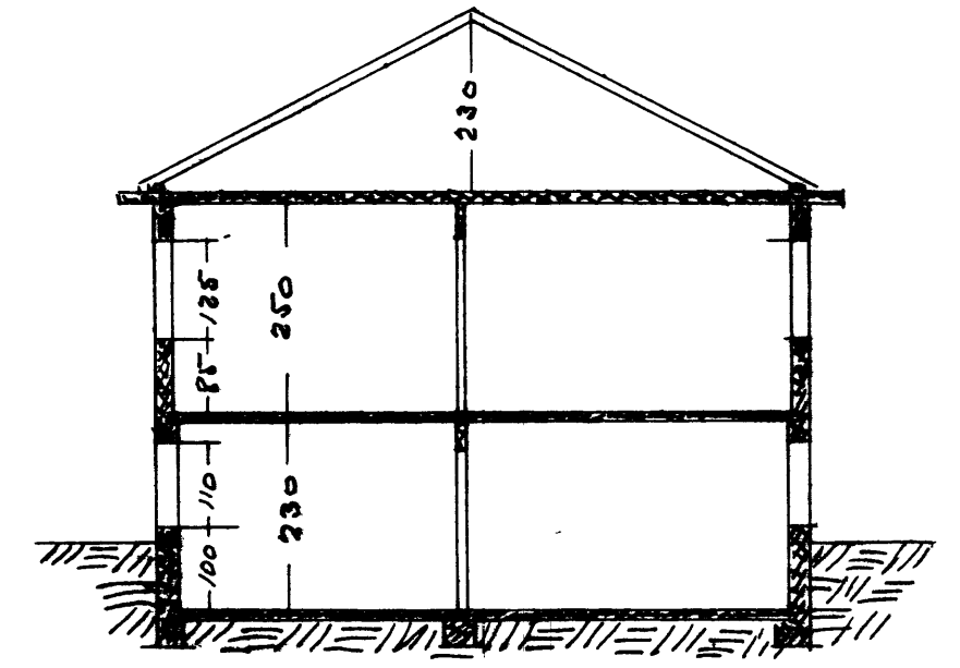
SKURÐUR
