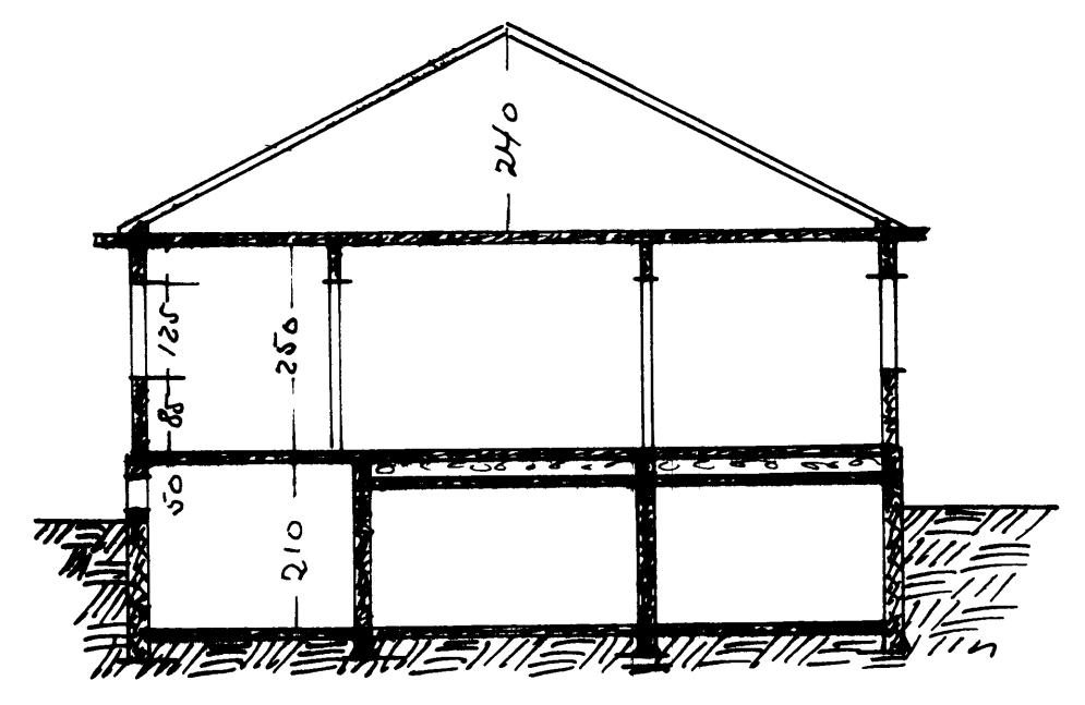
SKURÐUR
