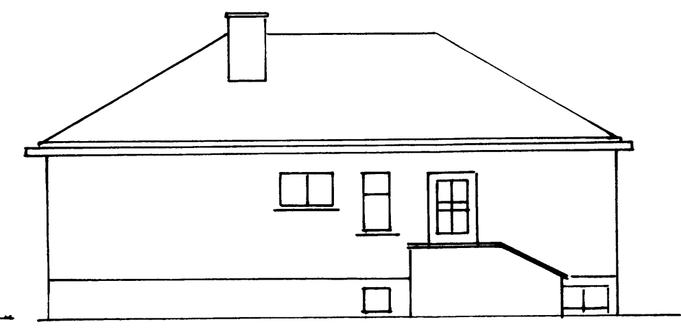
AUSTUR
