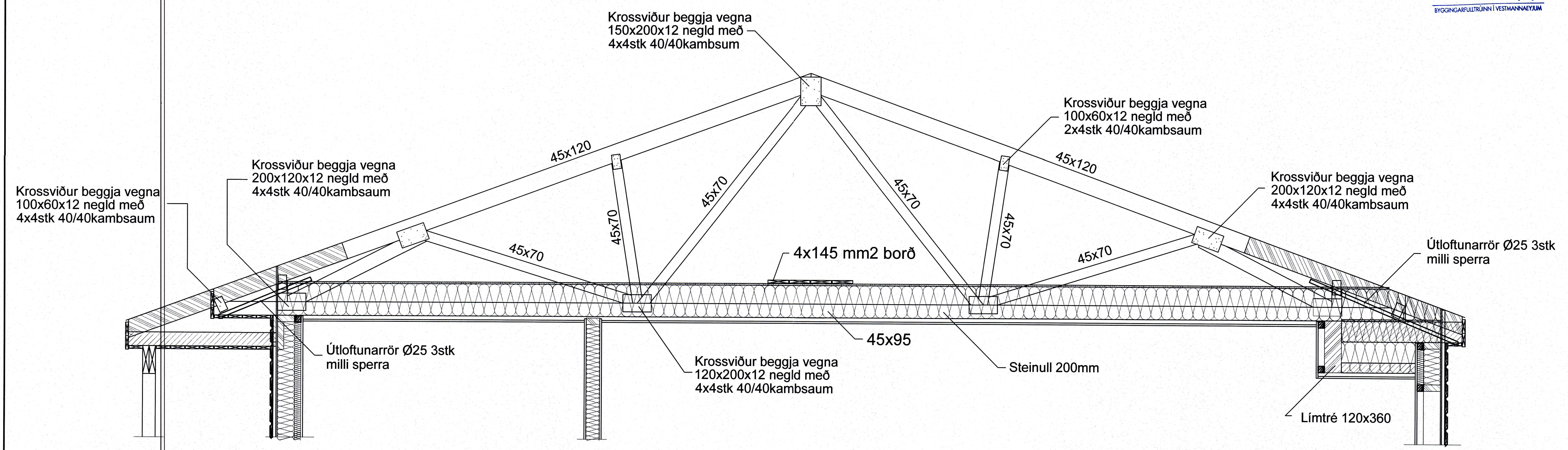
Hliðarmynd Mkv. 1:20
