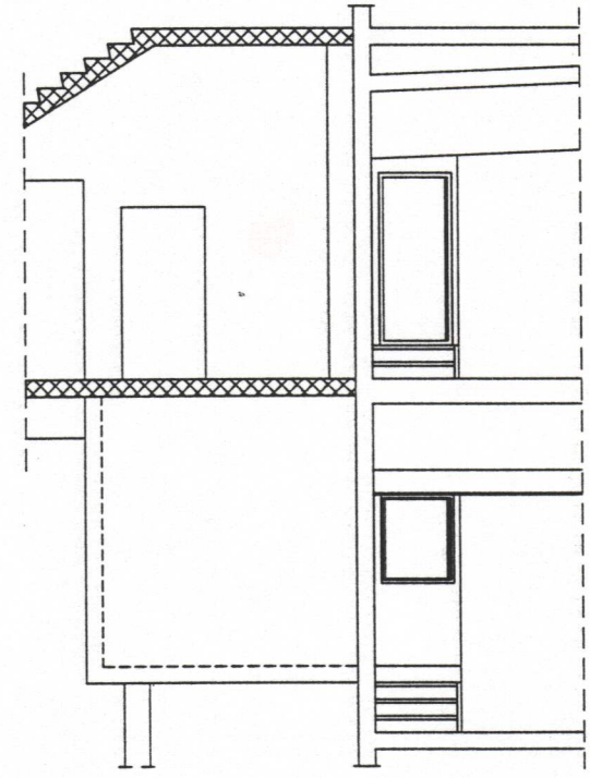
ÚTLIT HLIÐ
