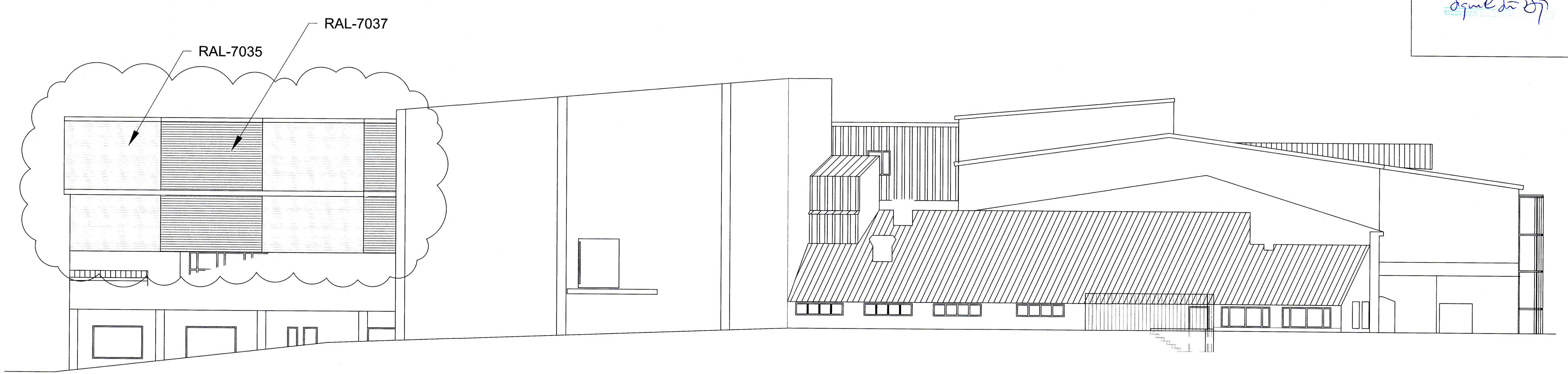
SUÐURHLIÐ Mkv: 1:100
