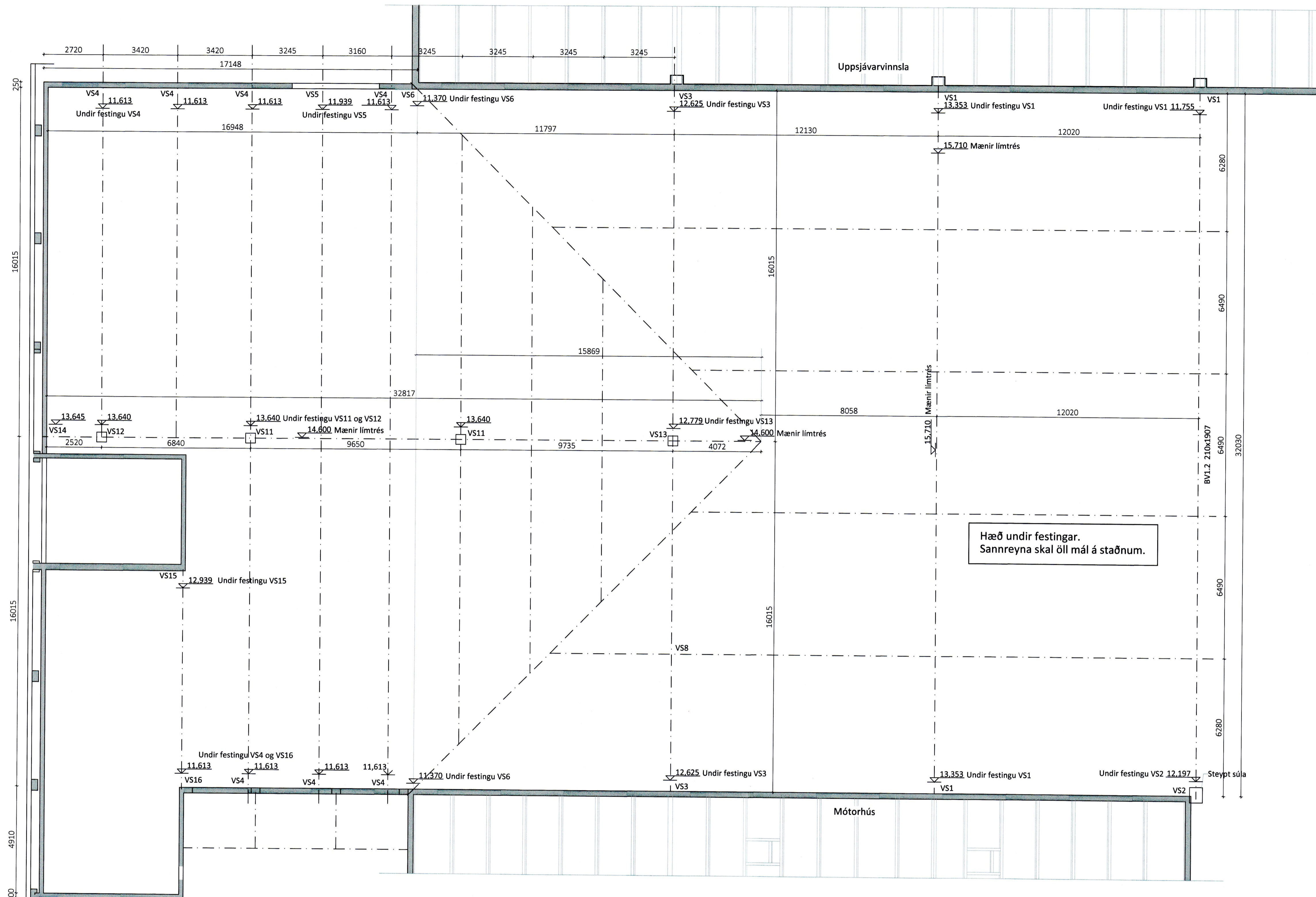
Þakmynd Mkv. 1:100 Hæð undir festingar
