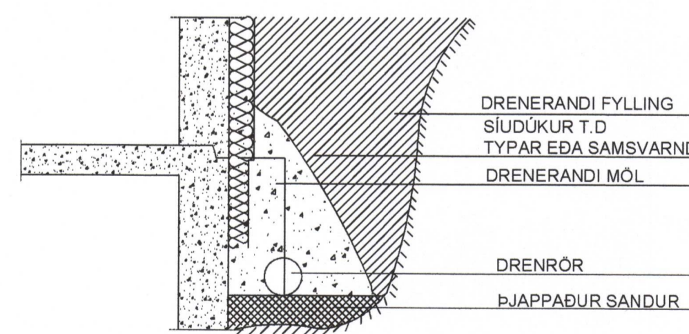
FRÁGANGUR DRENLAGNAR
