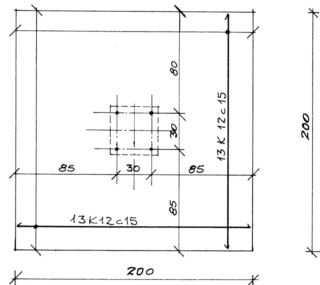
UNDIRSTAÐA U1 1:20.
