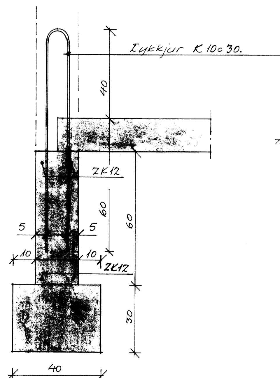
A-A 1:10.
