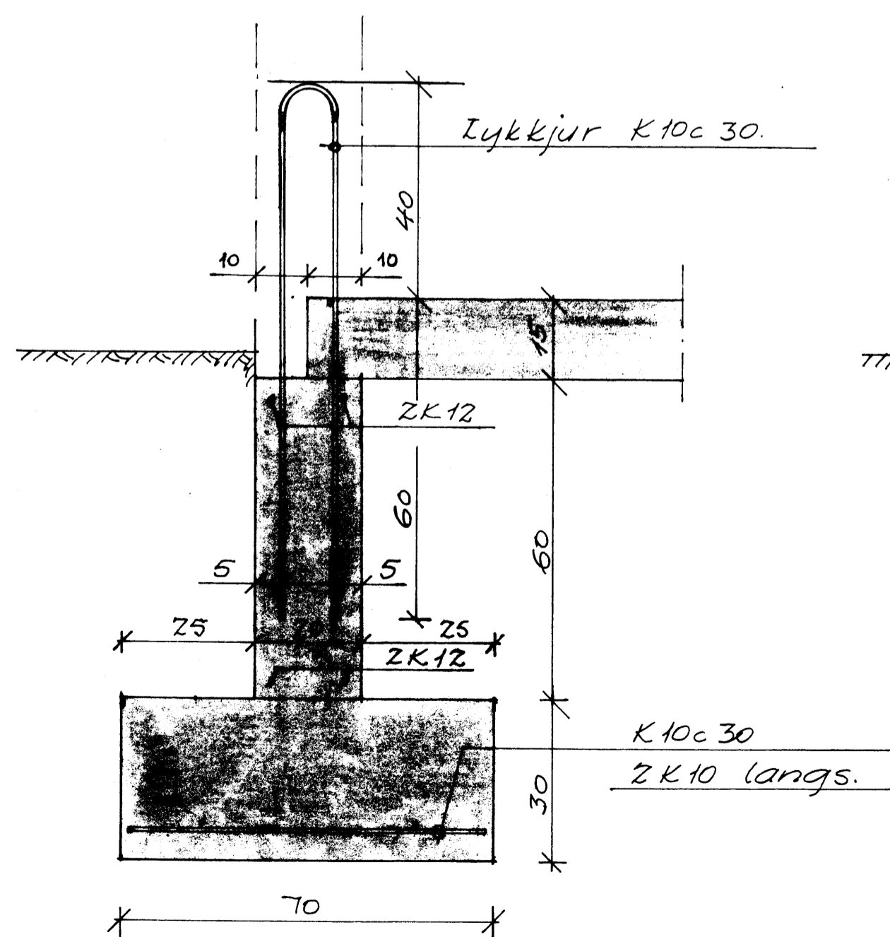
SNIÐ Í ÚTVEGGJASÖKKUL 1:10.
