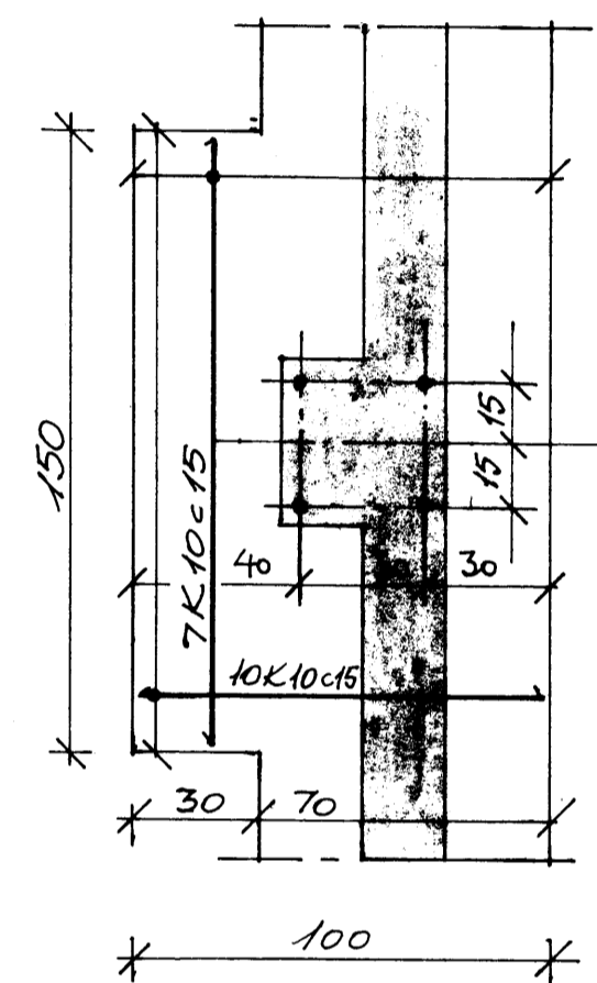
UNDIRSTAÐA U2 1:20.
