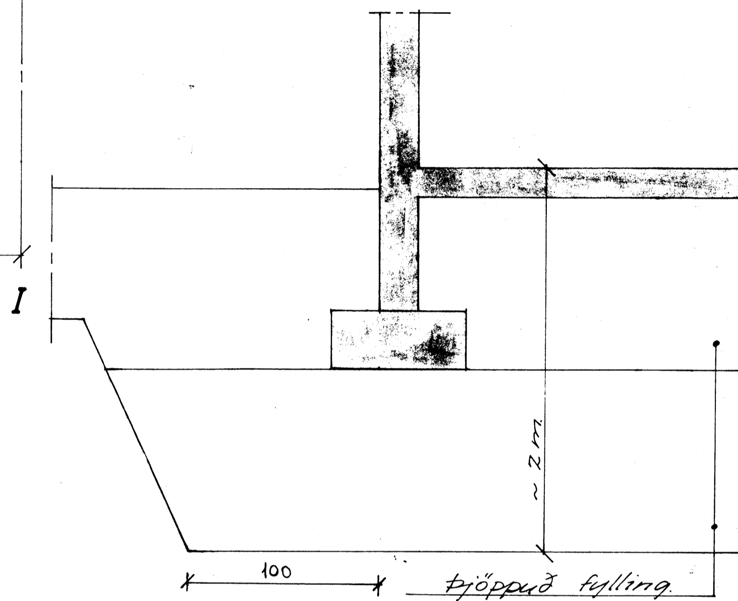
SNIÐ Í FYLLINGU 1:20.
