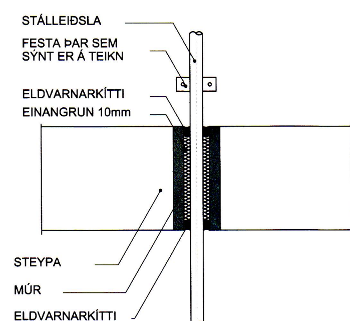
FRÁGANGUR Á STÁLLEIDSLU GEGNUM STEYPT GÓLF
