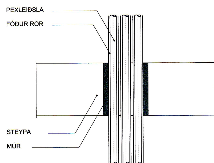
FRÁGANGUR Á PEKLEIDSLU GEGNUM STEYPT GÓLF
