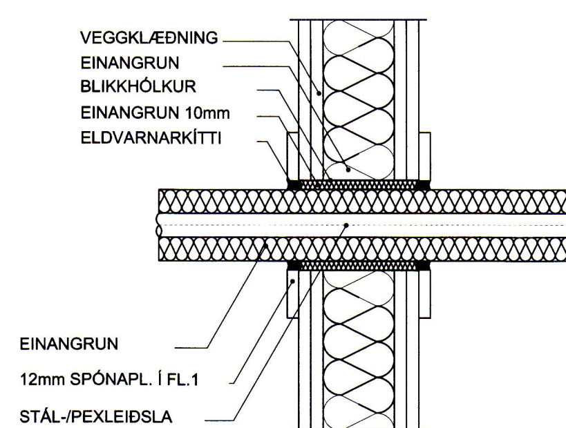
FRÁGANGUR Á STÁL-/PEKLEIDSLU GEGNUM LÉTTAN VEGG
