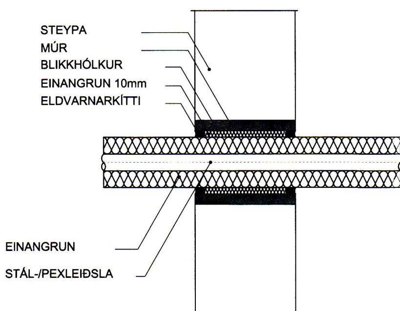
FRÁGANGUR Á STÁL-/PEKLEIDSLU GEGNUM STEYPTAN VEGG
