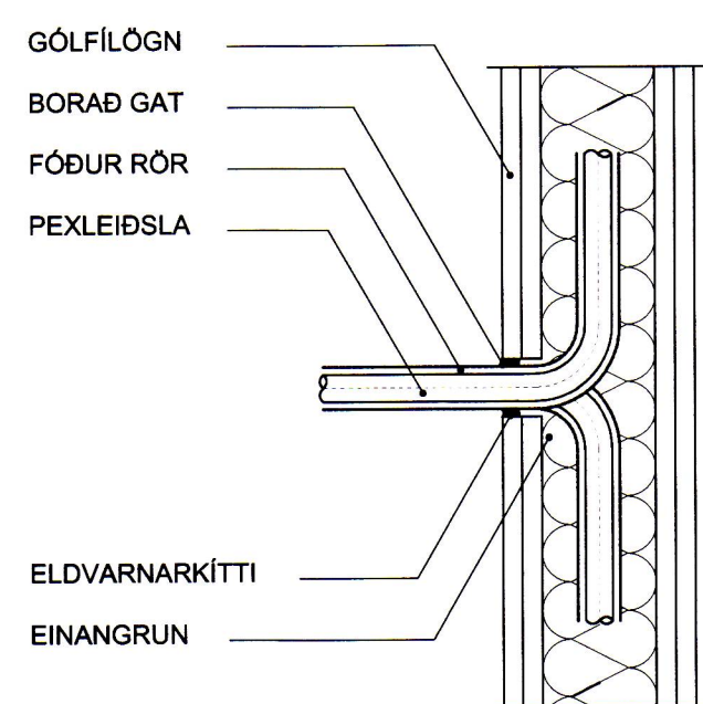
BRUNAPÉTTING Á PEKLEIDSLU Í FÓÐURRÖRI Í GEGNUM KLÆÐNINGU
