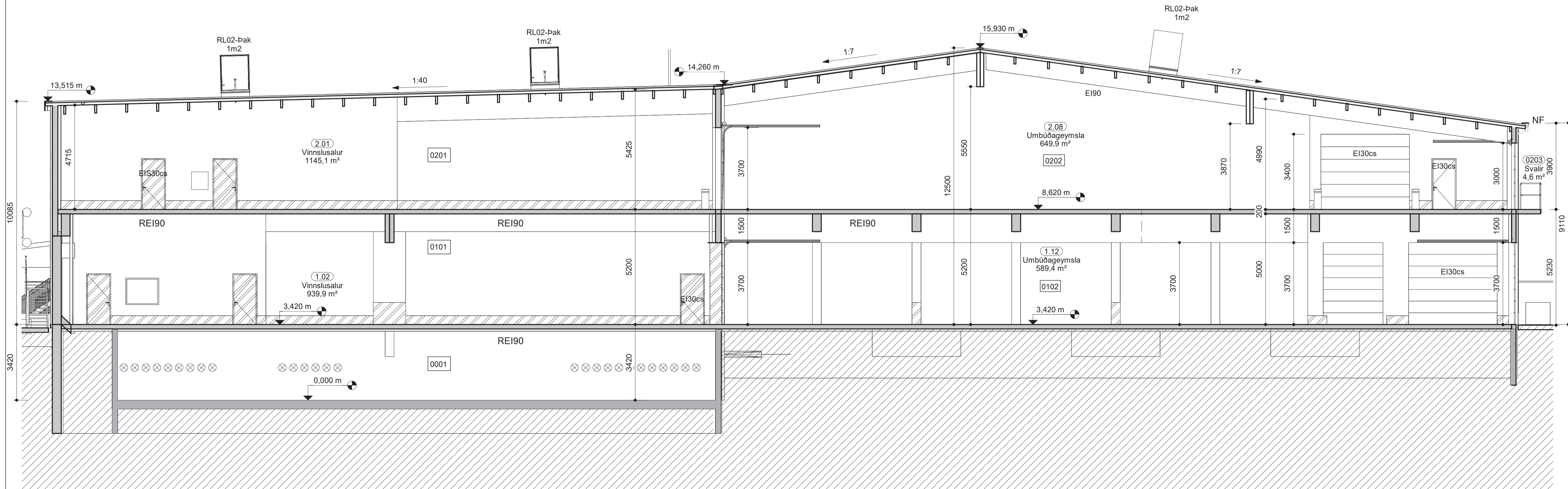
BB langsnið umbúðageymsla. mkv: 1 : 100
