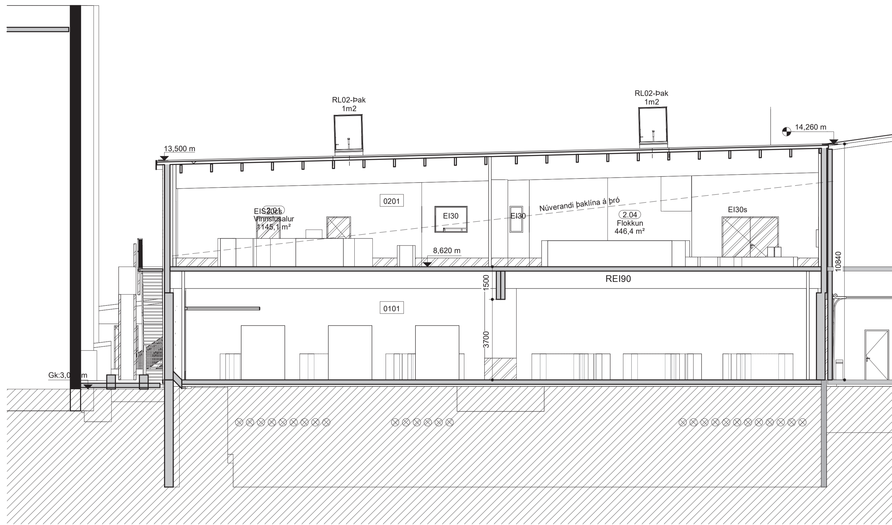
AA þversnið þró. mkv: 1 : 100
