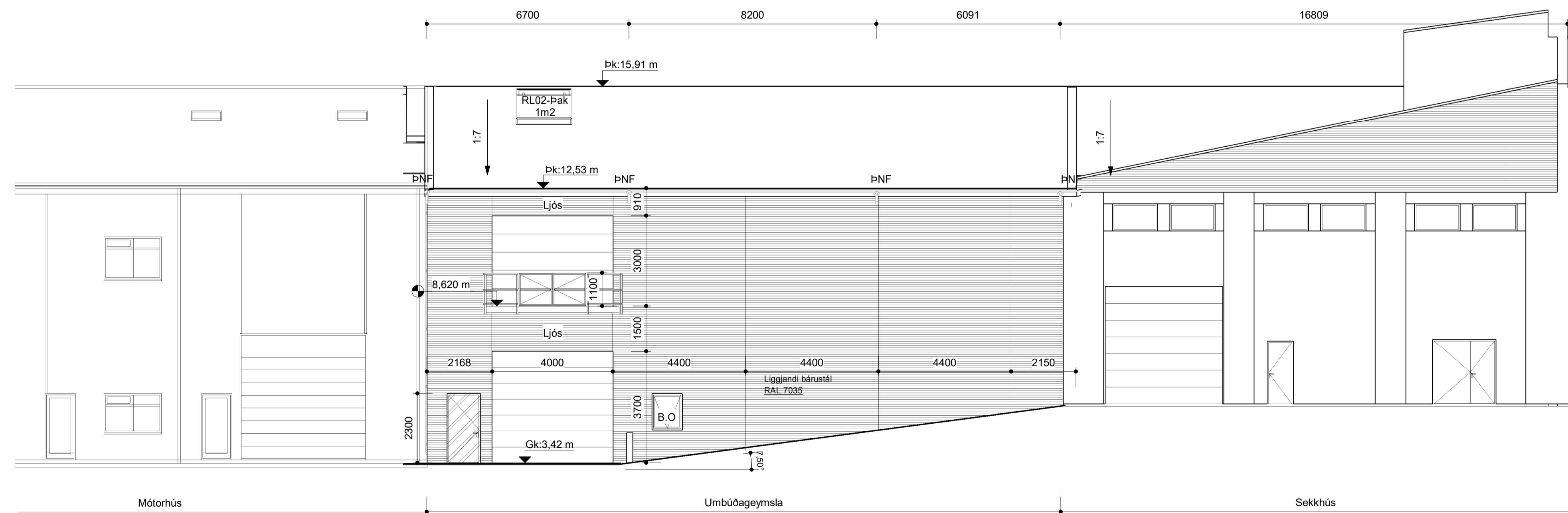
útlit vestur mkv: 1 : 100
