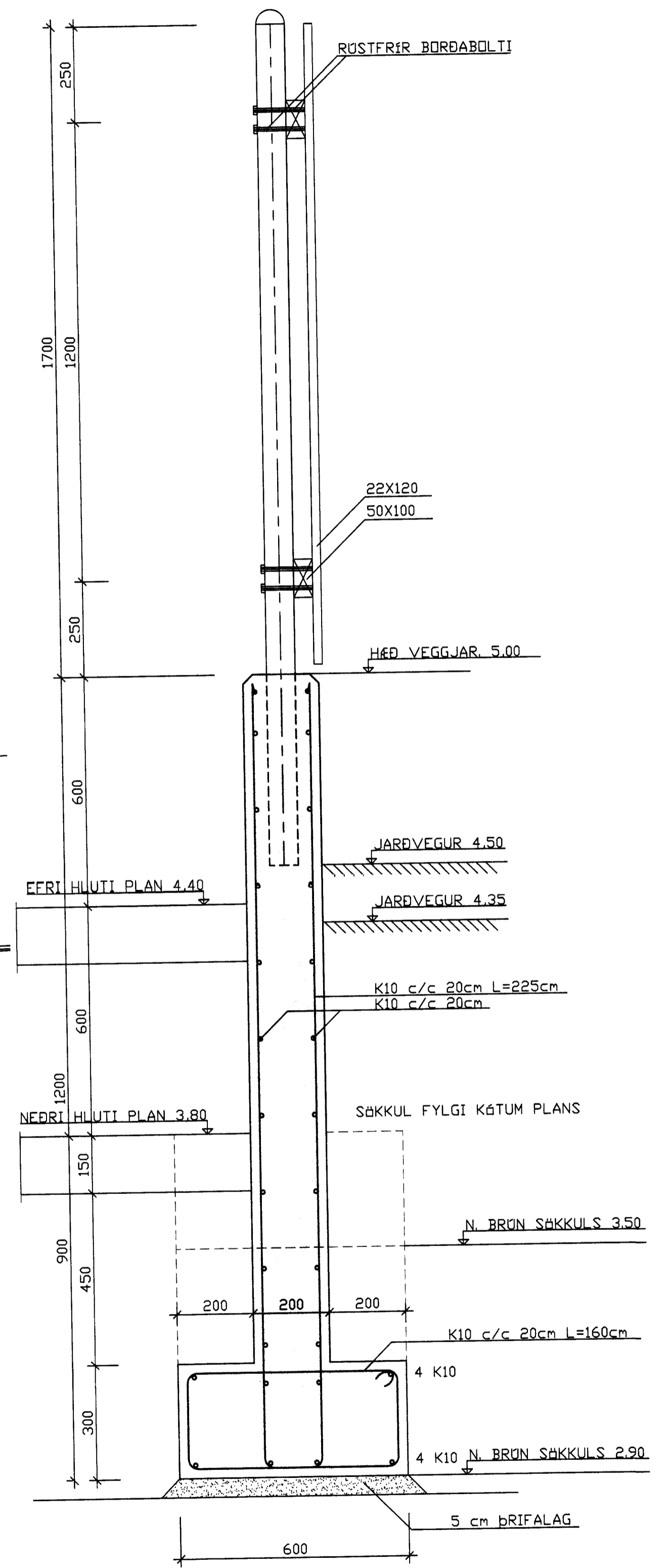
LÓÐRÉTT SNID M=1:10
