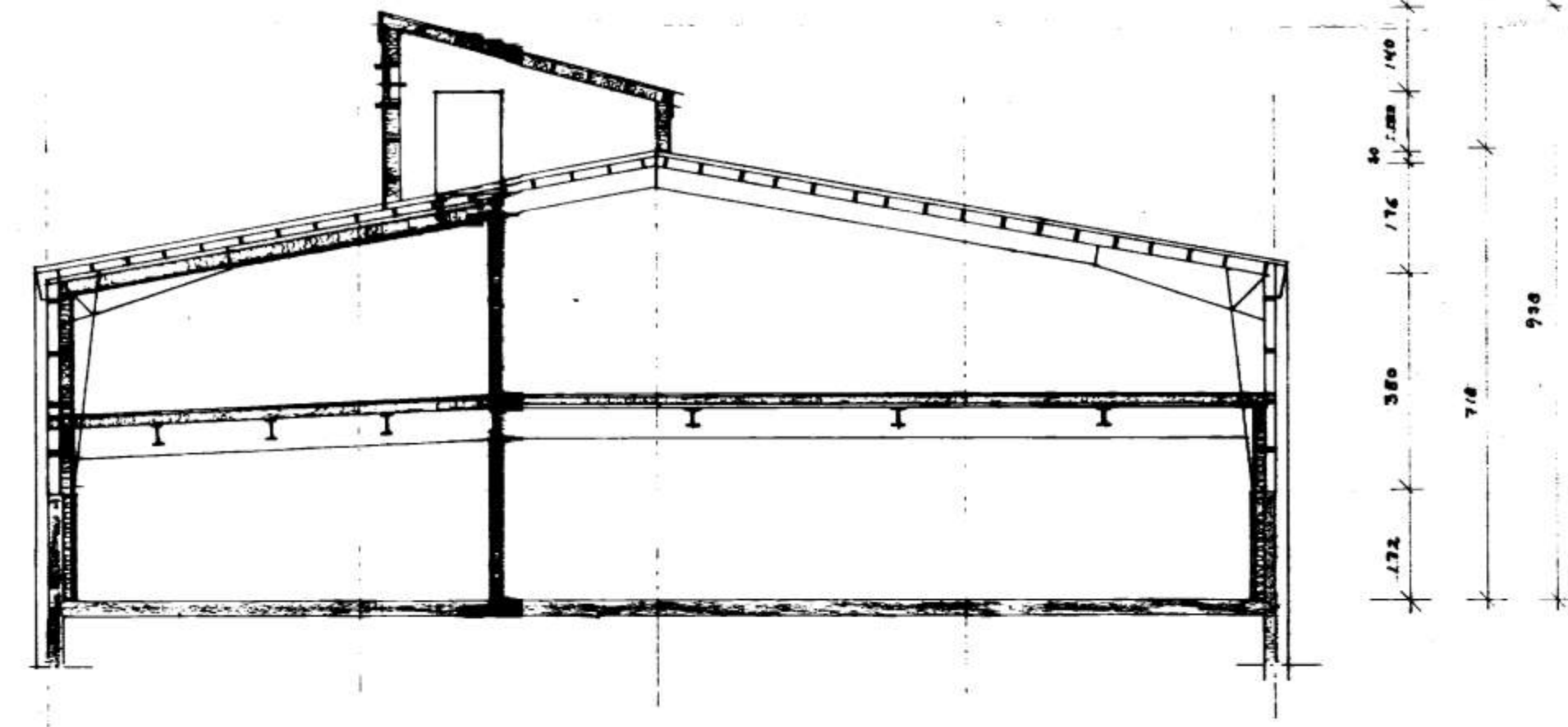
SNID A-A 1:100
