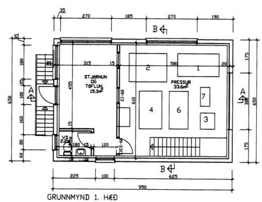
GRUNNMYND 1. HÆÐ
