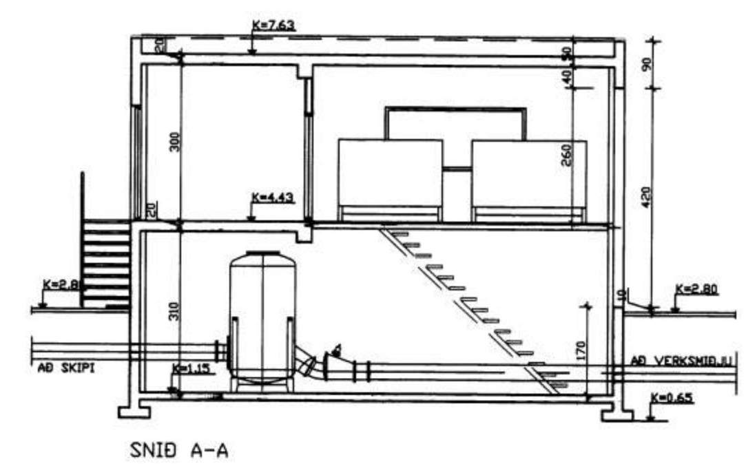
SNID A-A
