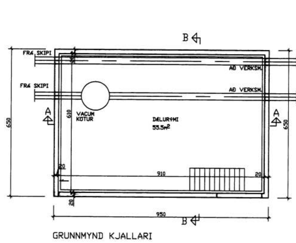
GRUNNMYND KJALLARI
