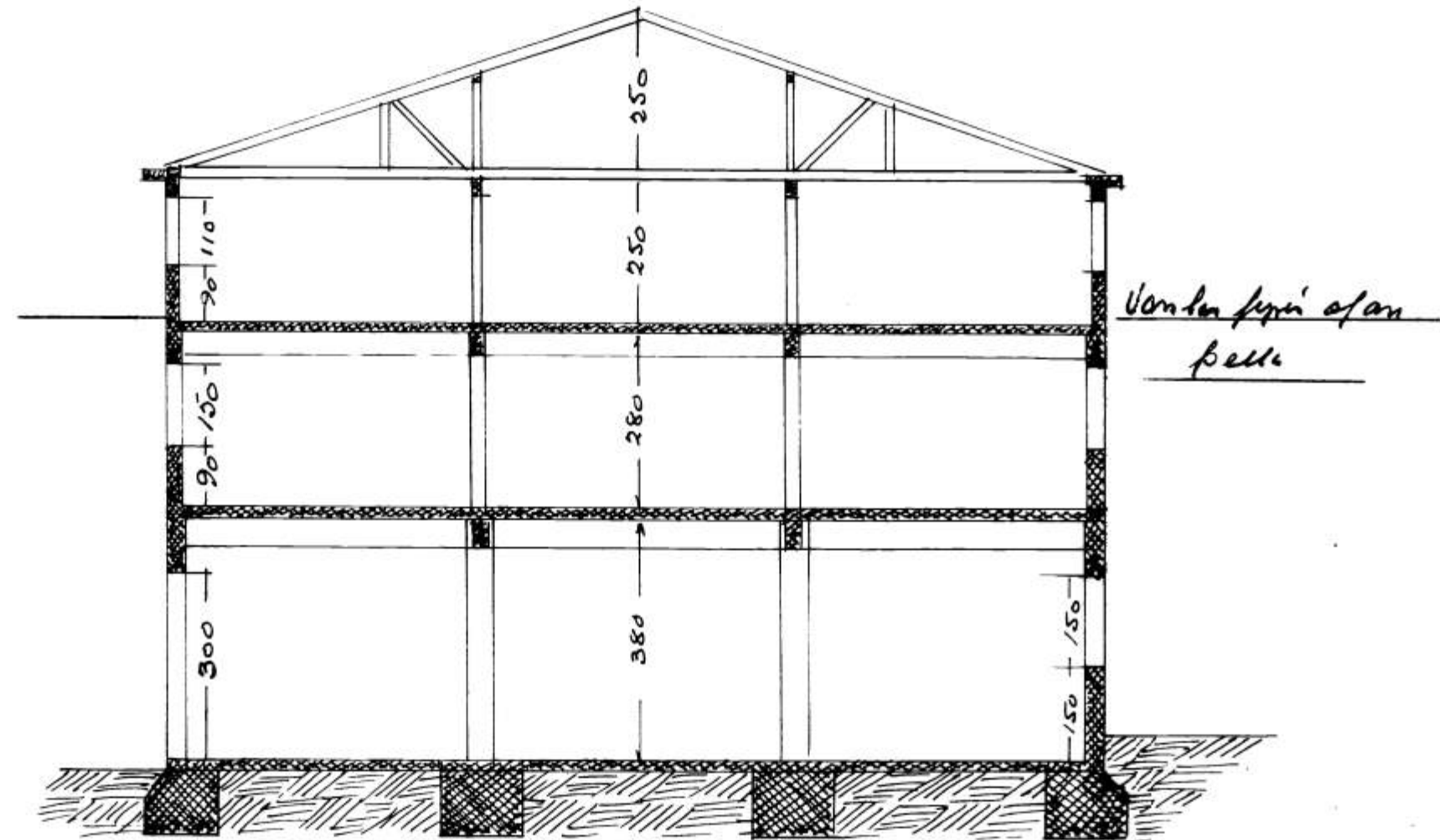
SKURÐUR
