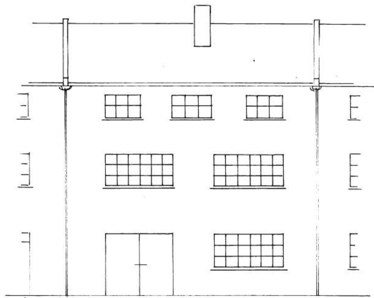
SÚÐUR
