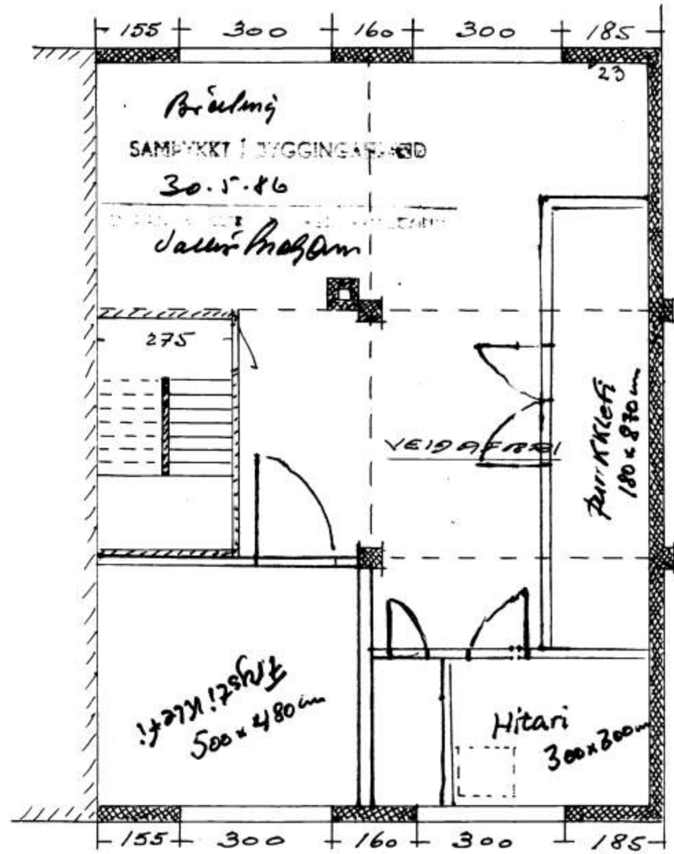
2. HÆÐ
