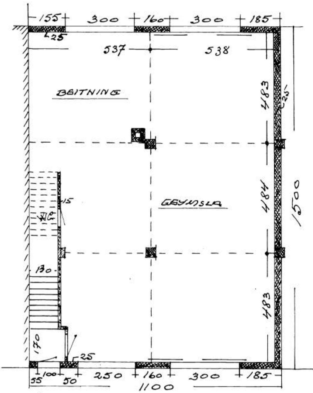
1. HÆÐ
