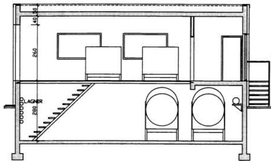
SNID A-A
