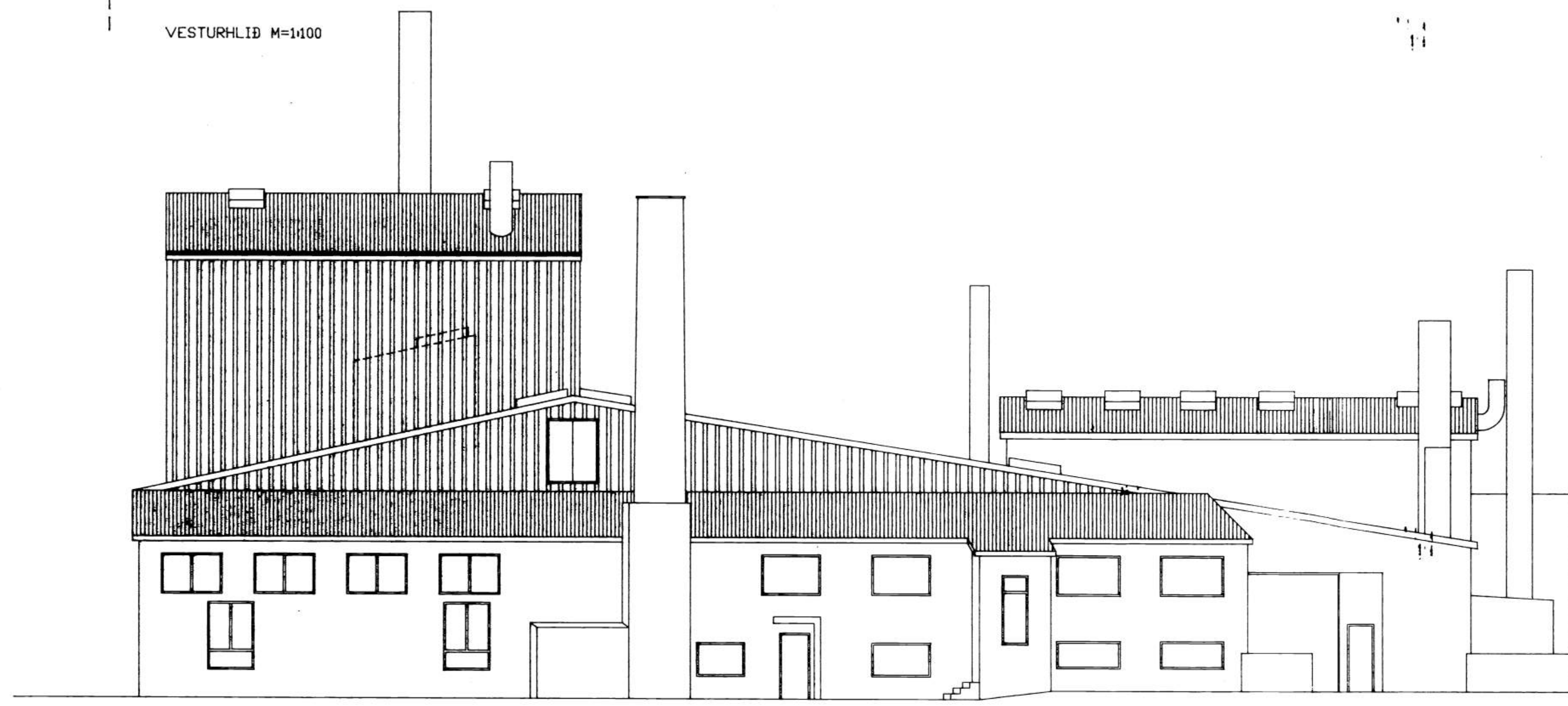
SUÐURHLIÐ M=1:100
