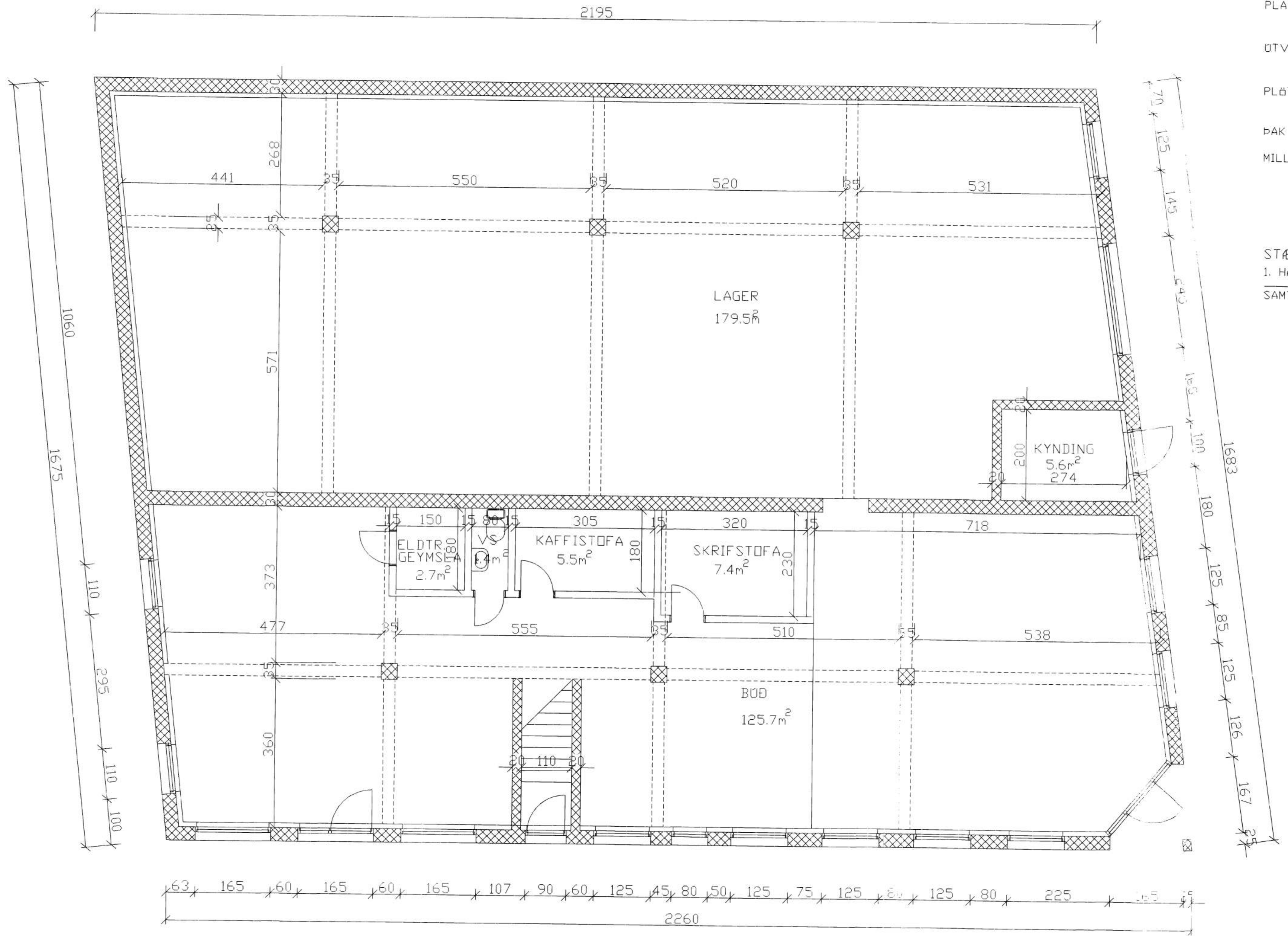
GRUNNMYND 1 HÆÐ M=1:50
