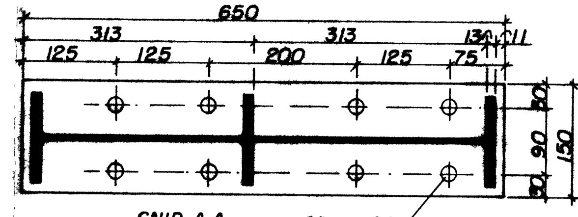
SNIP A-A MKV 1:5
