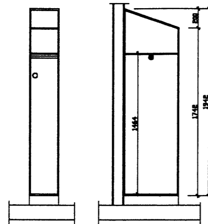
STARFSMANNASKAPAR 6 STK M=120
