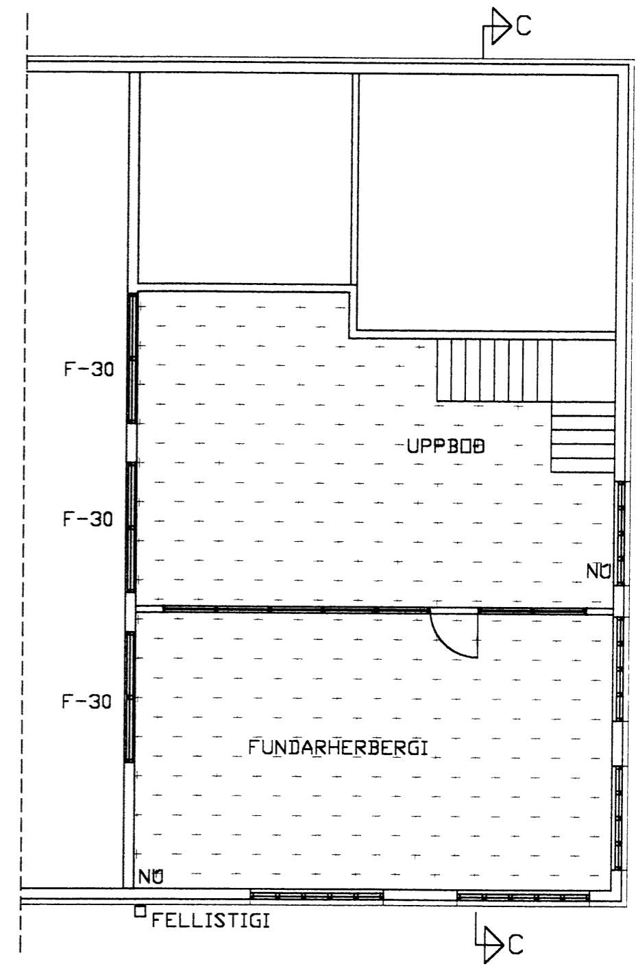
GRUNNMYND 2. HÆÐ
