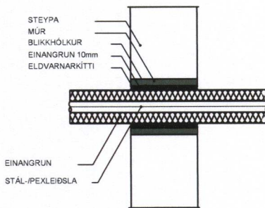
FRÁGANGUR Á STÁL-/PEXLEIÐSLU GEGNUM STEYPTAN VEGG
