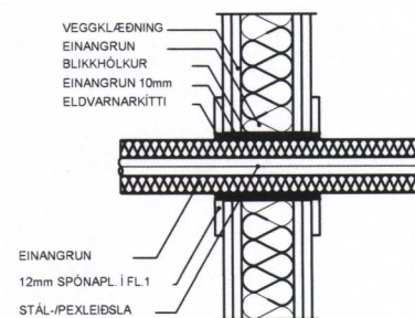
FRÁGANGUR Á STÁL-/PEXLEIÐSLU GEGNUM LÉTTAN VEGG
