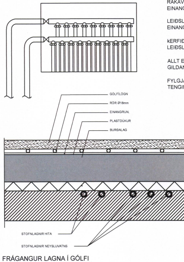
FRÁGANGUR LAGNA Í GÓLFI
