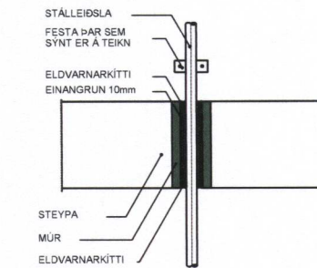
FRÁGANGUR Á STÁLLEIÐSLU GEGNUM STEYPT GÓLF
