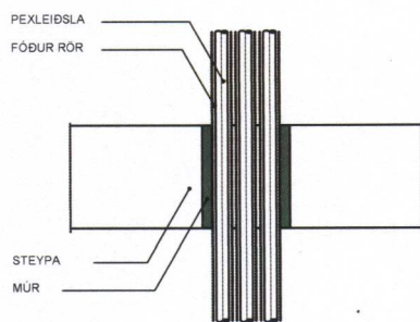
FRÁGANGUR Á PEXLEIÐSLU GEGNUM STEYPT GÓLF
