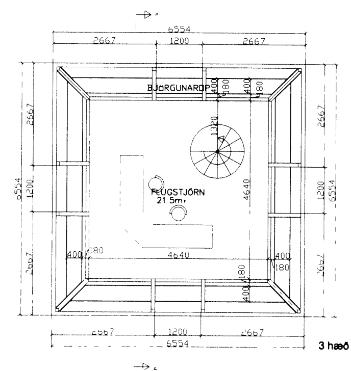
3 hæð
