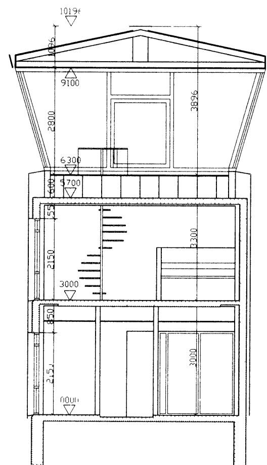
Sneiðing AA
