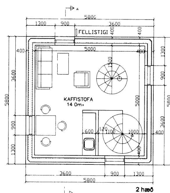
2 hæð
