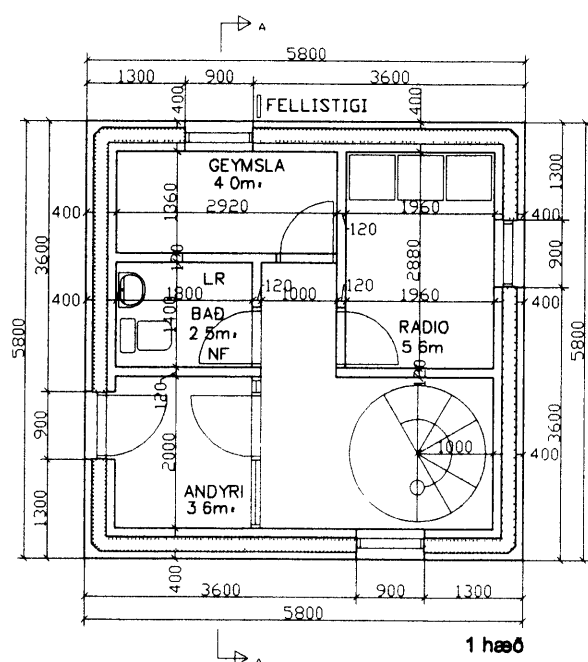
1 hæð
