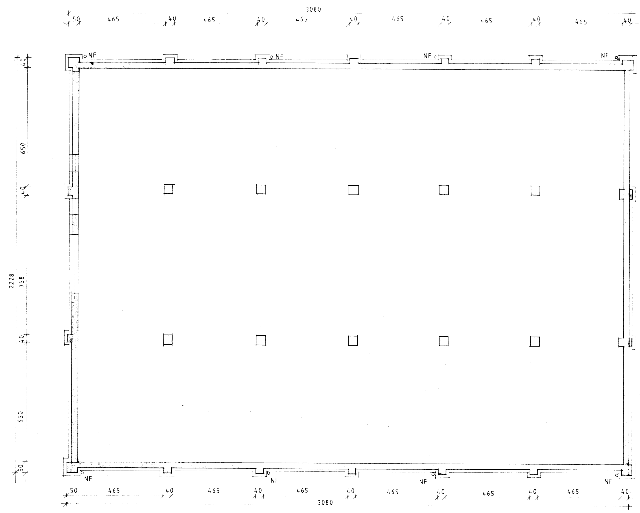
GRUNNMYND 1. HÆÐ M=1:100
