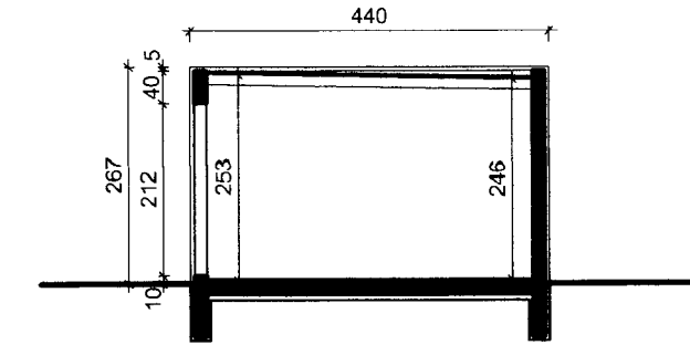
Snið A-A 1:100
