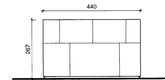
Útlit austur 1:100
