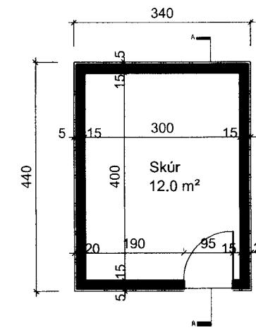
Grunnmynd 1:100
