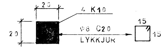
SÚLA 3, 1:20
