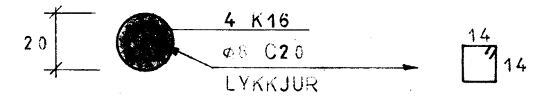
SÚLA 1, 1:20
