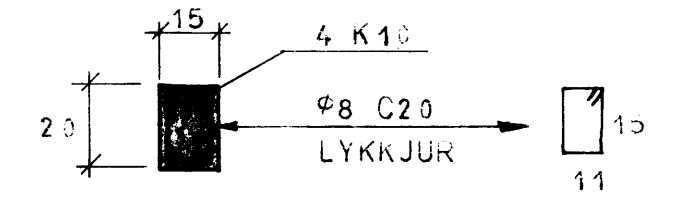
SÚLA 4, 1:20
