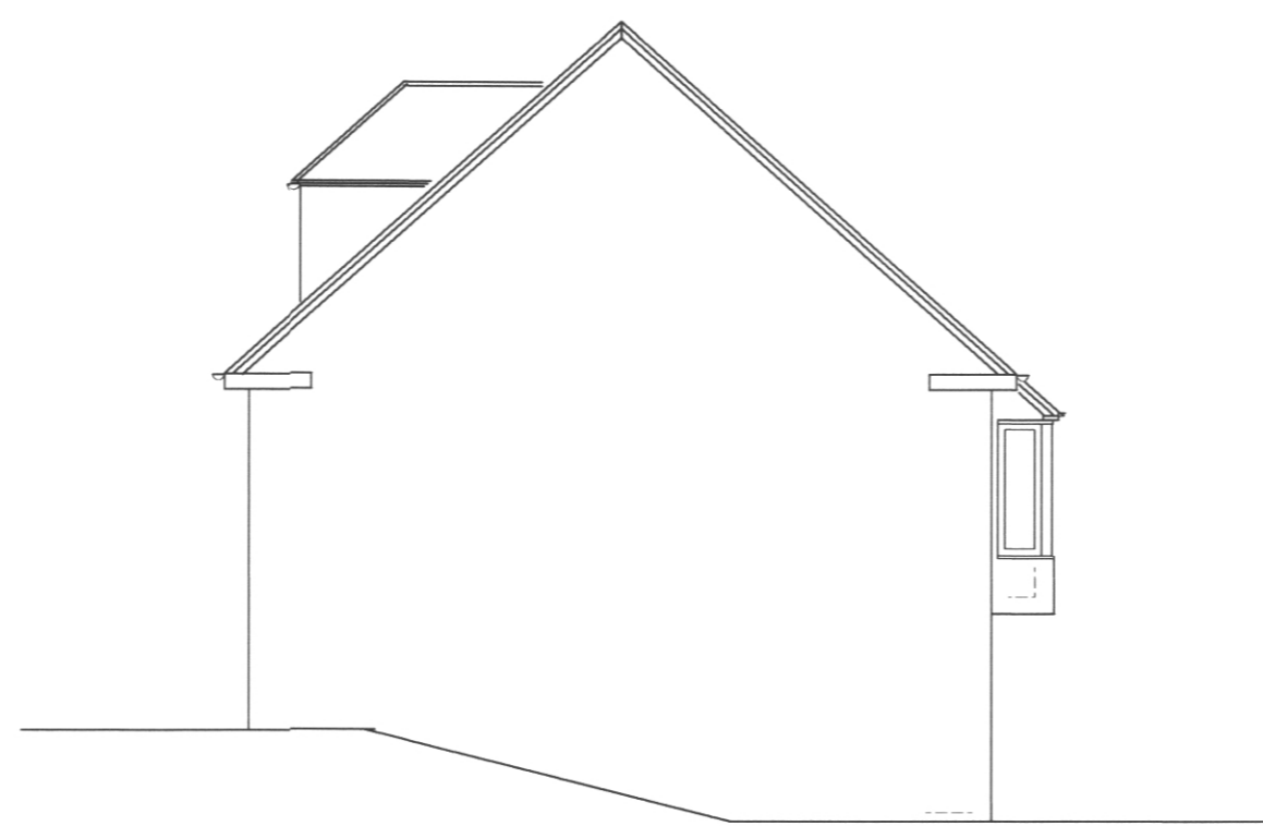
- AUSTUR mkv. 1 : 100
