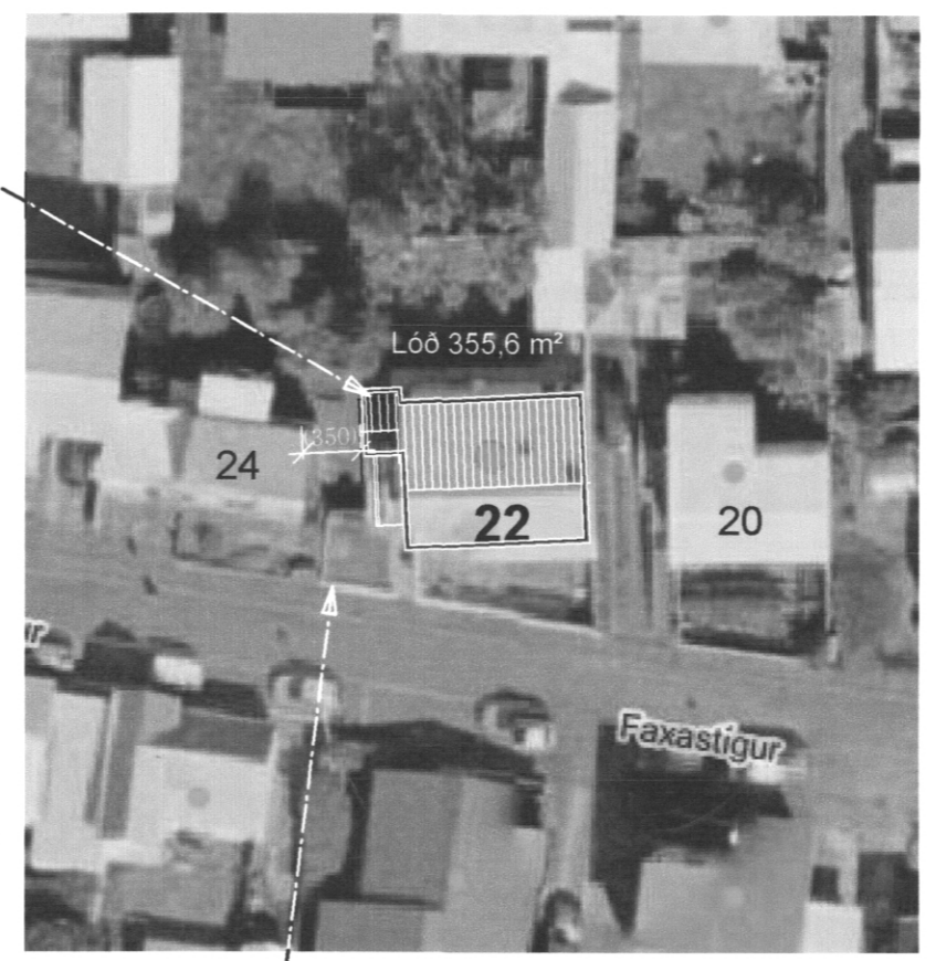
AFSTÖÐUMYND mkv. 1 : 500
