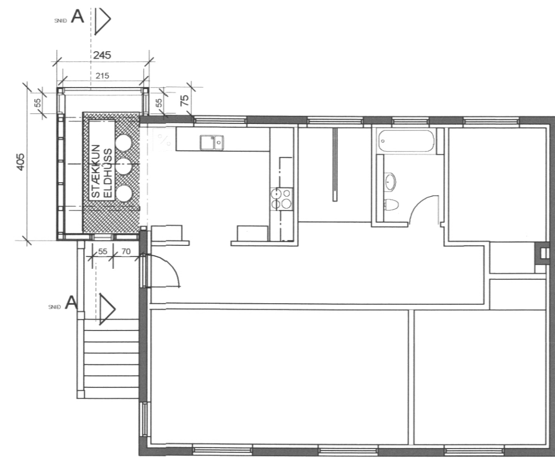
GRUNNMYND 1 : 100
