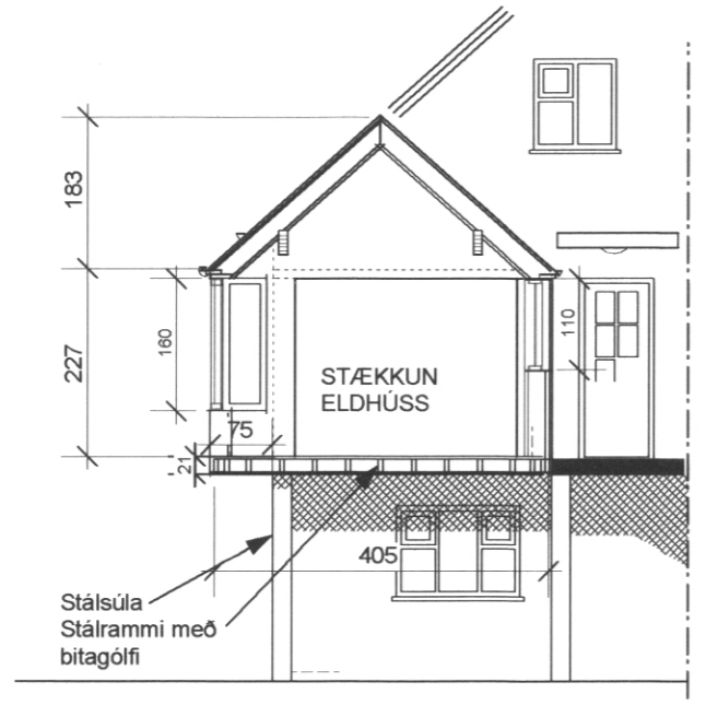
- VESTUR mkv. 1 : 100
