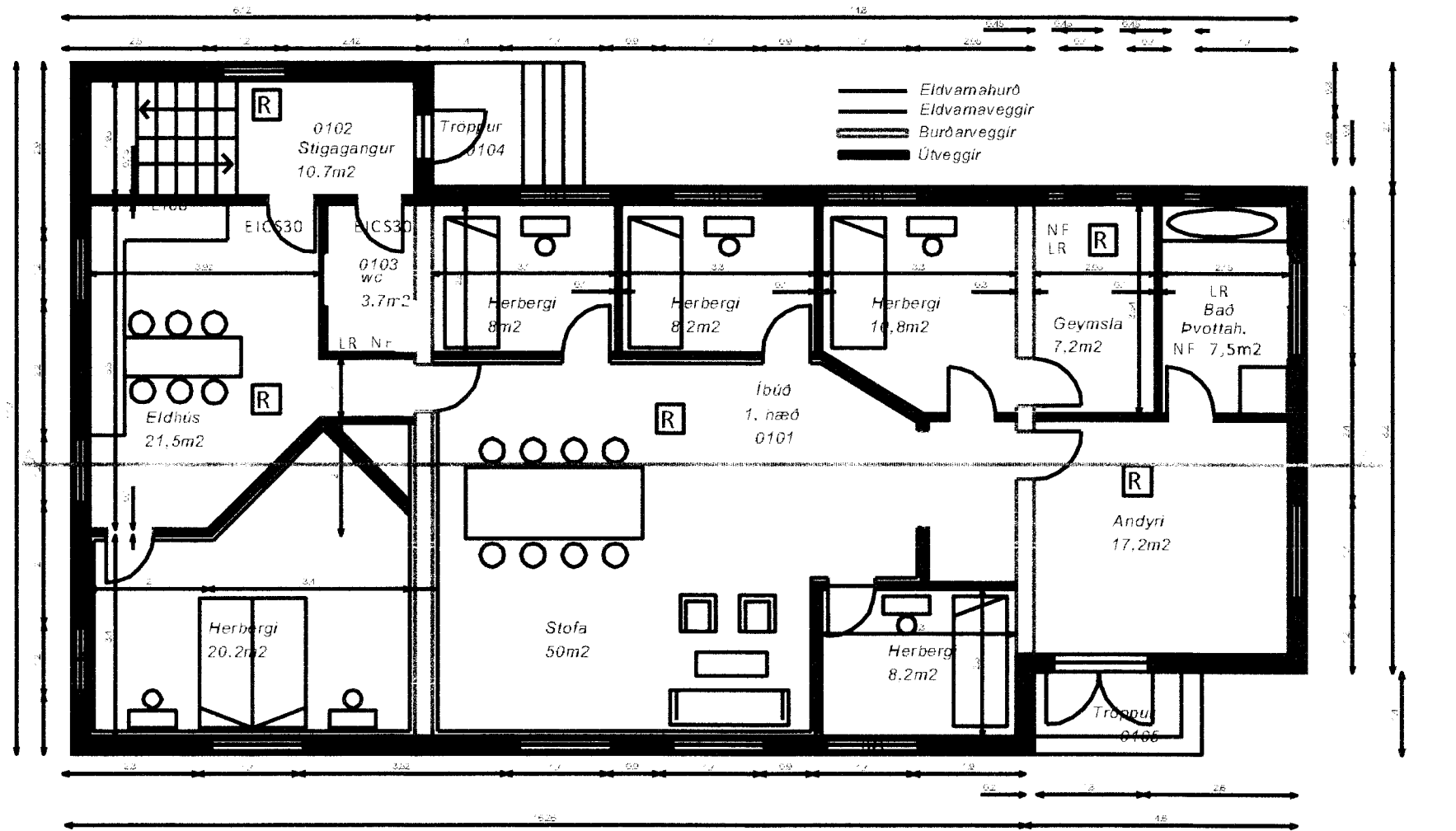
Grunnmynd 1. hæð Mkv. 1:100
