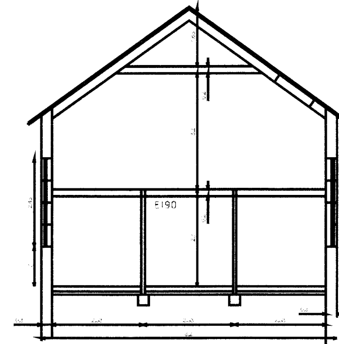
Þversnið B-B Mkv. 1:100
