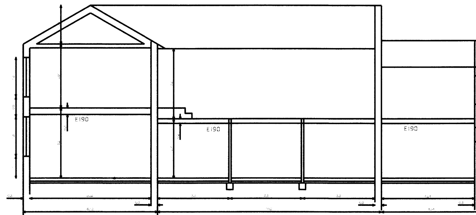
Langsnið A-A Mkv. 1:100
