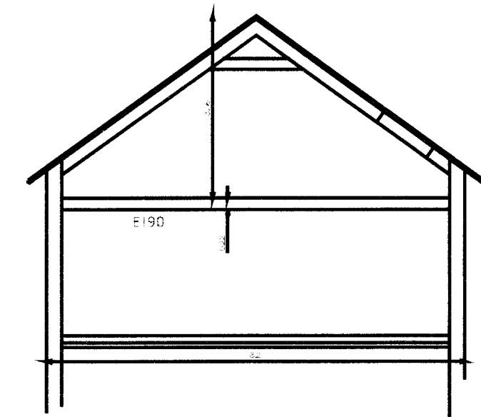
Þversnið C-C Mkv. 1:100
