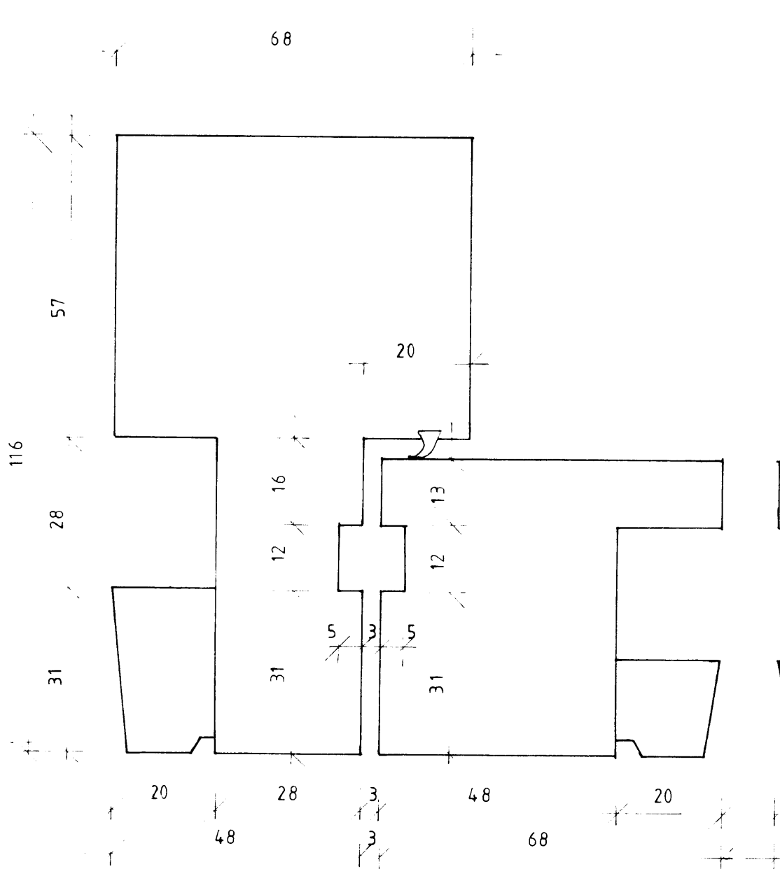
MILLISTYKKI FÖST RÚÐA VINSTRA MEGIN OPNALEGT FAG HÆGRA MEGIN
