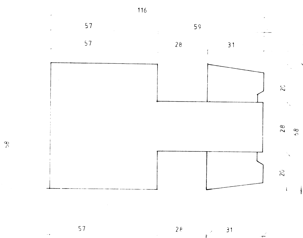
MILLISTYKKI FÖST RÚÐA BÄÐUM MEGIN
