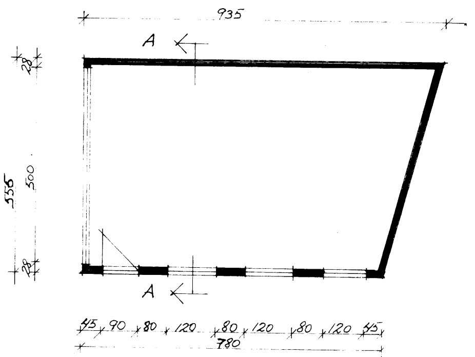
GRUNNMYND
