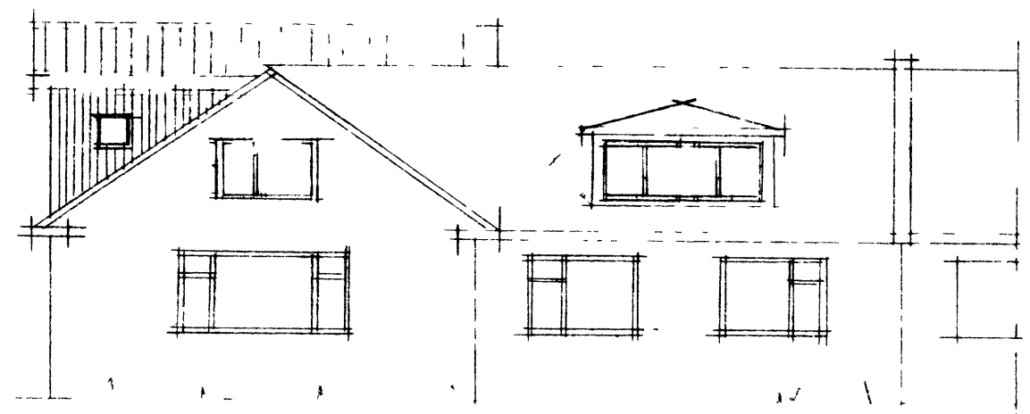
SÚÐURHLÍÐ
