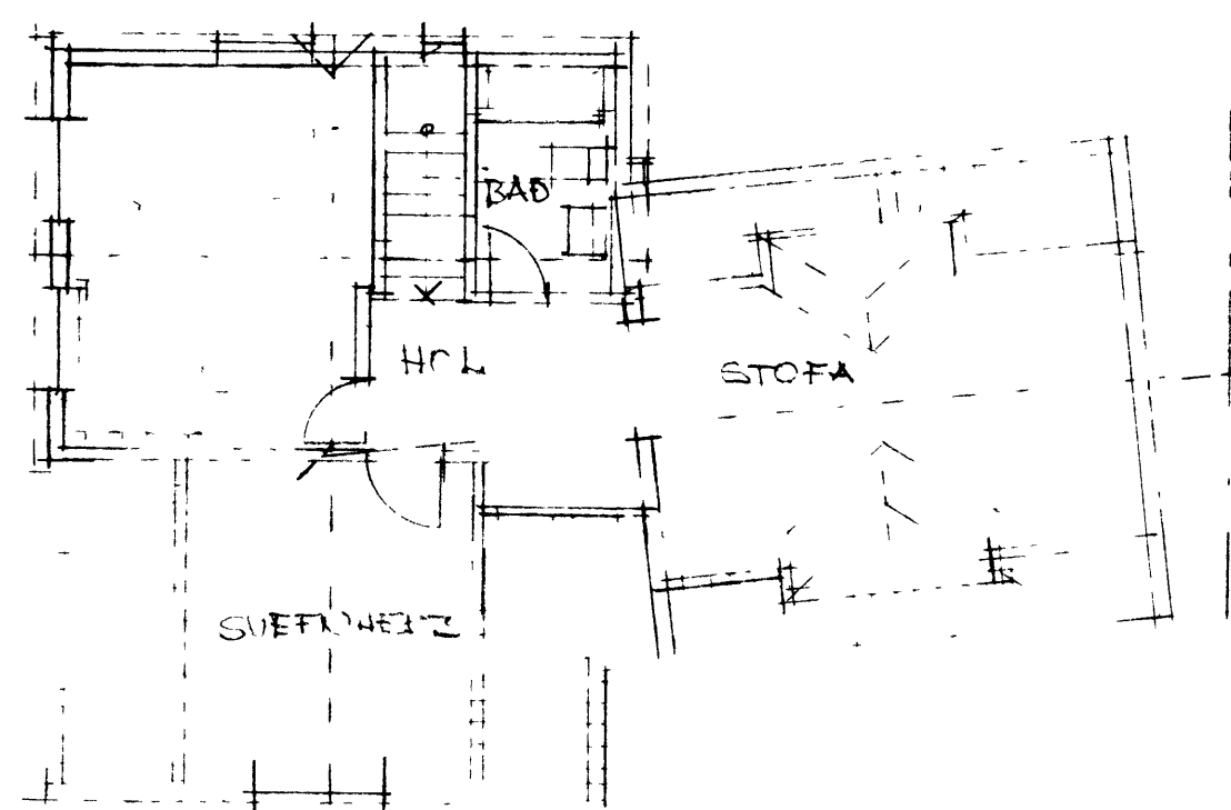
GRUNNMYND 2HÆÐ
