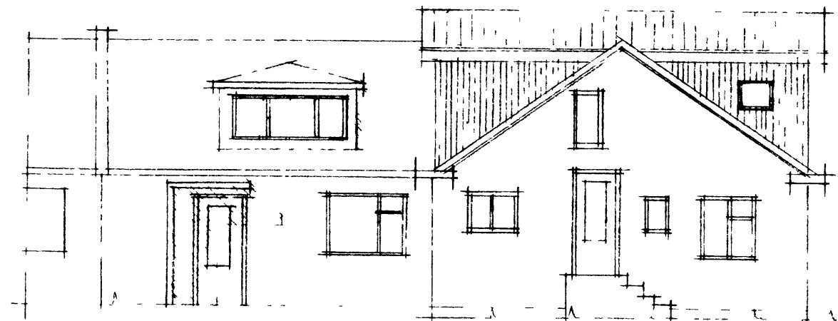
NOÐRURHLÍÐ
