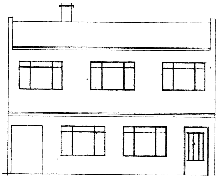
Framhlið M 1:100
