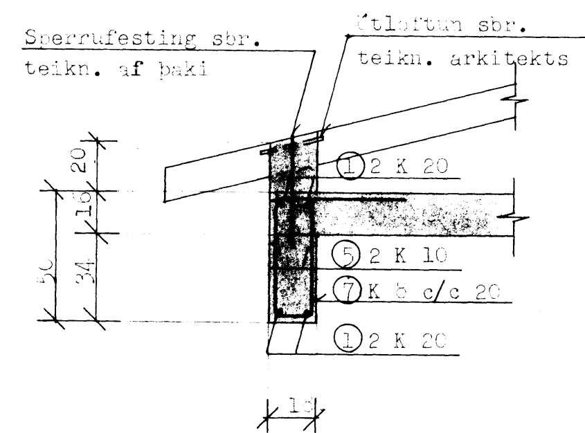
SNIÐ A-A 1:20
