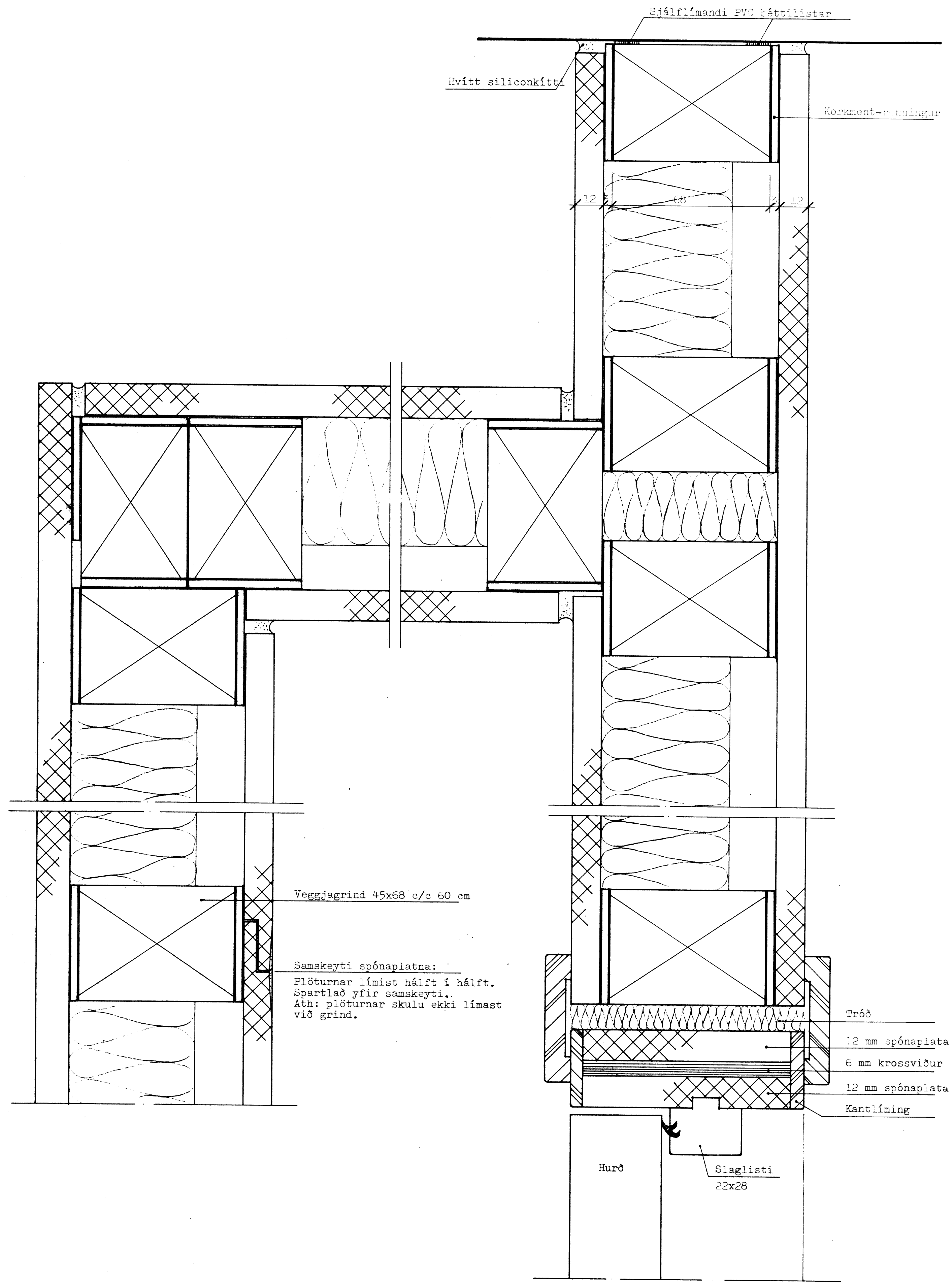
LÁRÉTTAR SNEIÐINGAR
