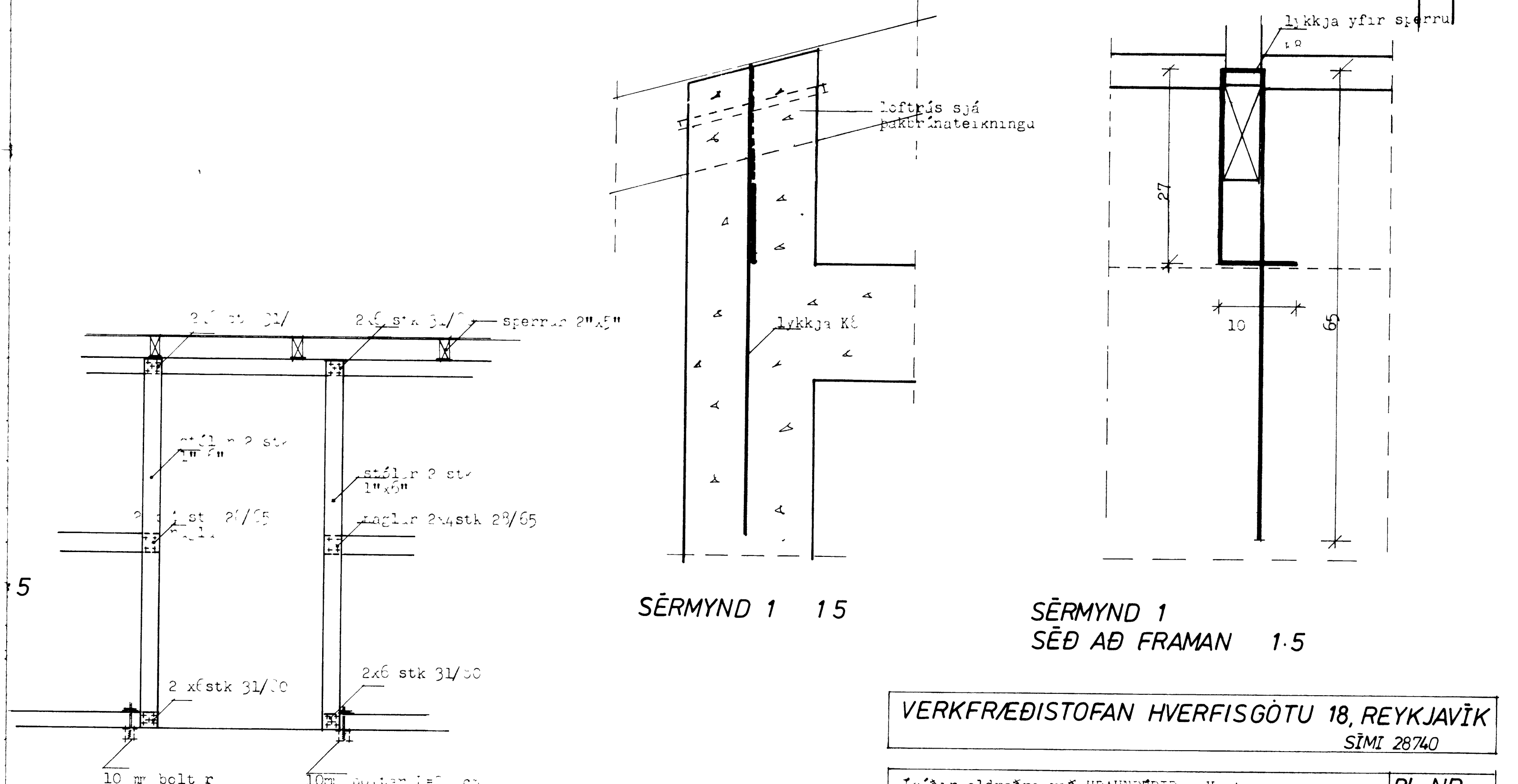
FRÁGANGUR VIÐ OP INN Í GEYMSLURÝMI 1:20
