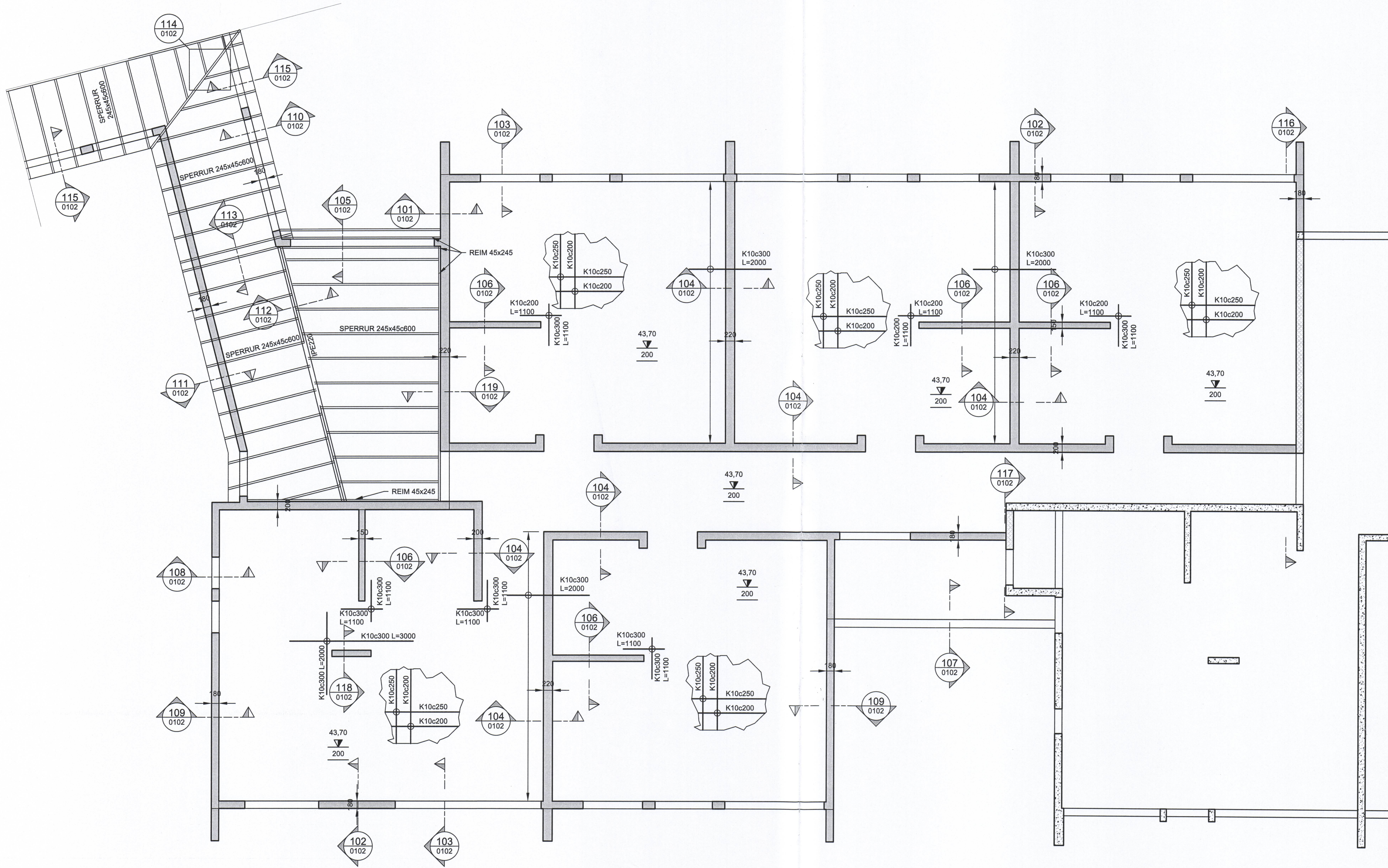
GRUNNMYND 1:50
