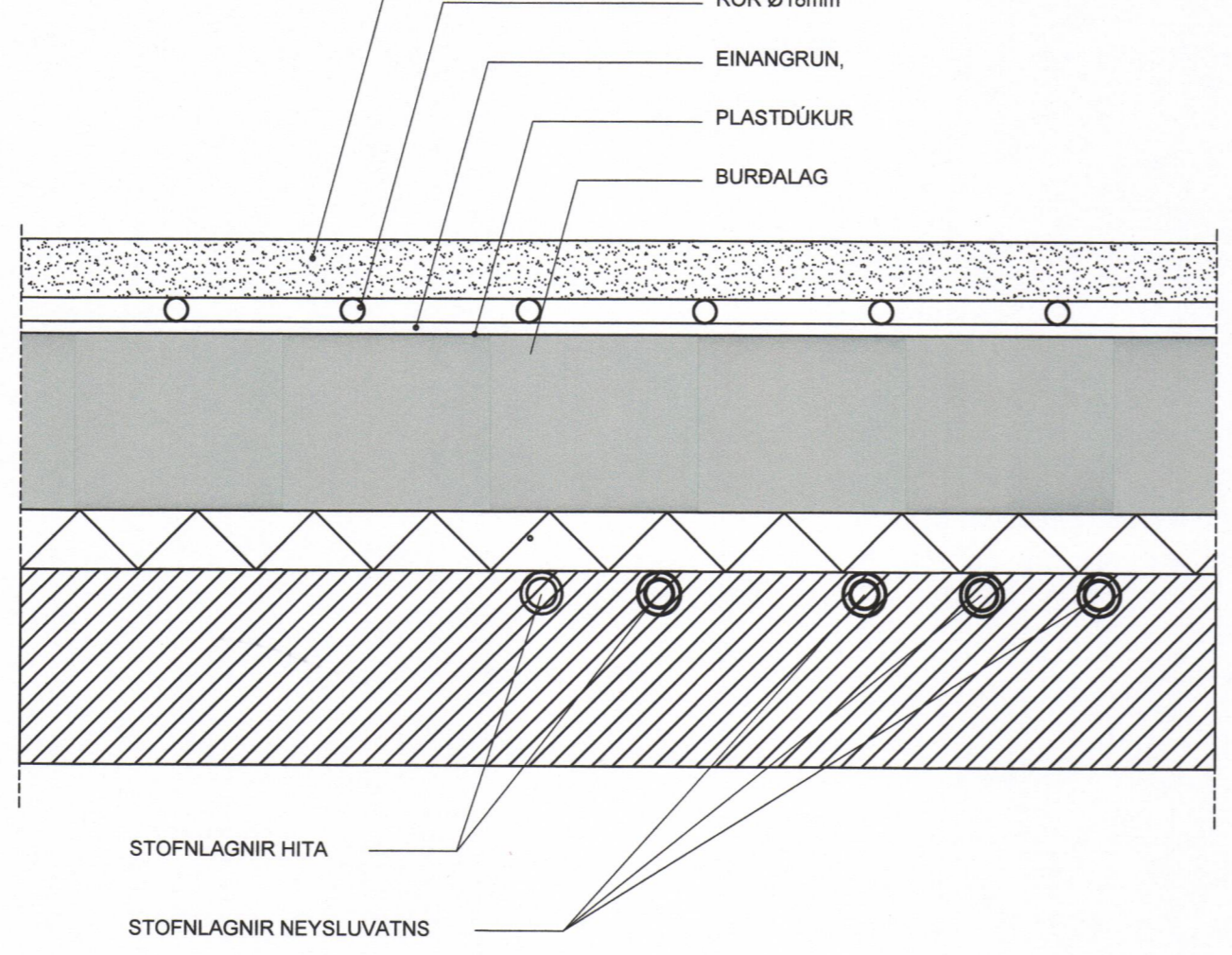
FRÁGANGUR LAGNA Í GÓLFI
