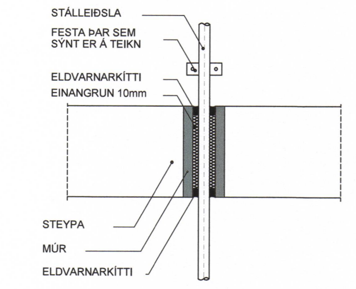
FRÁGANGUR Á STÁLLEISLU GEGNUM STEYPT GÓLF
