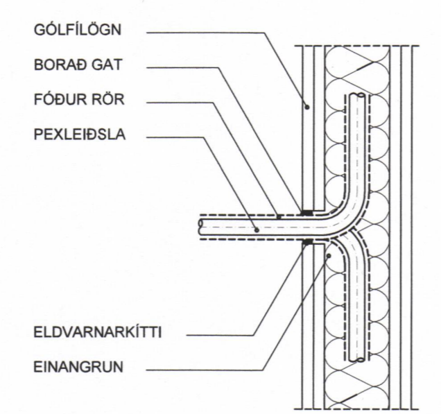
BRUNAPÉTTING Á PEKLEISLU Í FÓÐURRÖRI Í GEGNUM KLÆDNINGU
