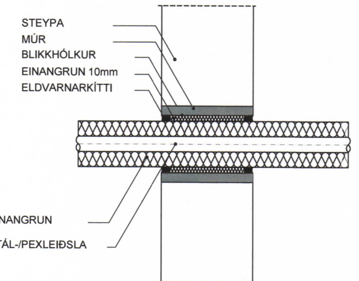
FRÁGANGUR Á STÁL-/PEKLEISLU GEGNUM STEYPTAN VEGG
