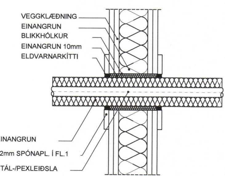
FRÁGANGUR Á STÁL-/PEKLEISLU GEGNUM LÉTTAN VEGG
