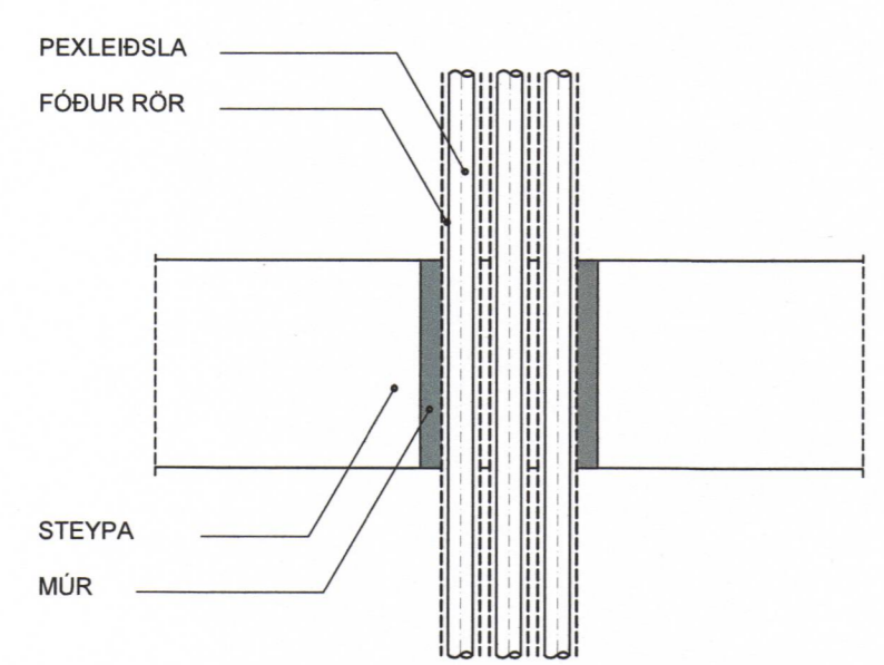
FRÁGANGUR Á PEKLEISLU GEGNUM STEYPT GÓLF
