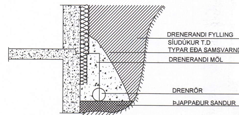
FRÁGANGUR DRENLAGNAR
